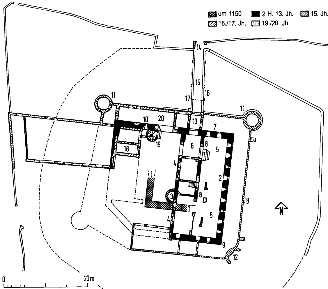
Abb. 11 Orschweier. Baualterplan mit Grabungsbefunden (Th. Biller, auf Grundlage des Grundrisses im Inventaire..., ct. Guebwiller).
