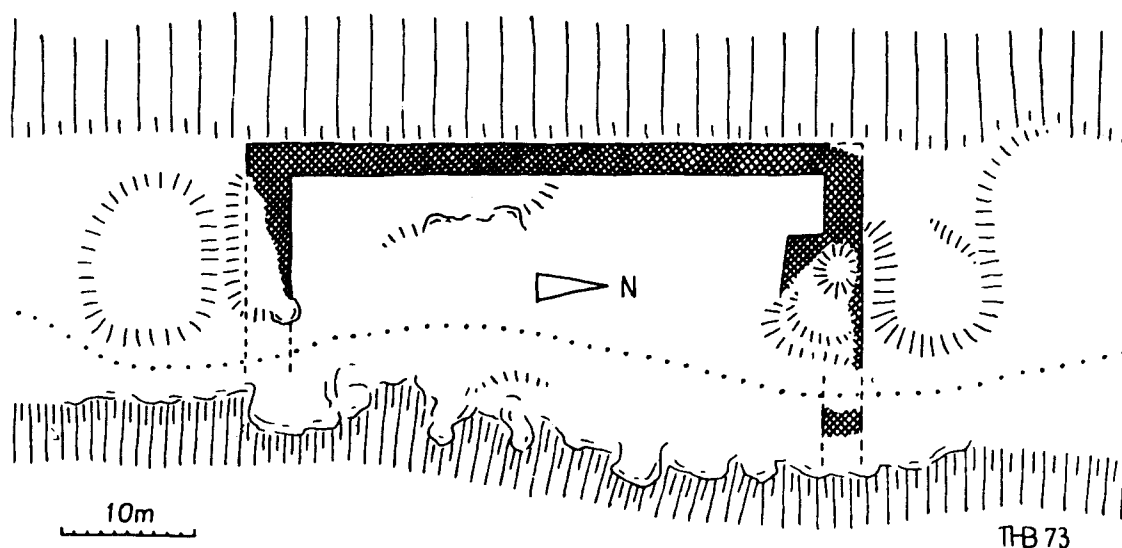
Abb. 8 Köpfel. Grundriß (Th. Biller, in: Archäol. Korrespondenzbl. 4, 1973).
