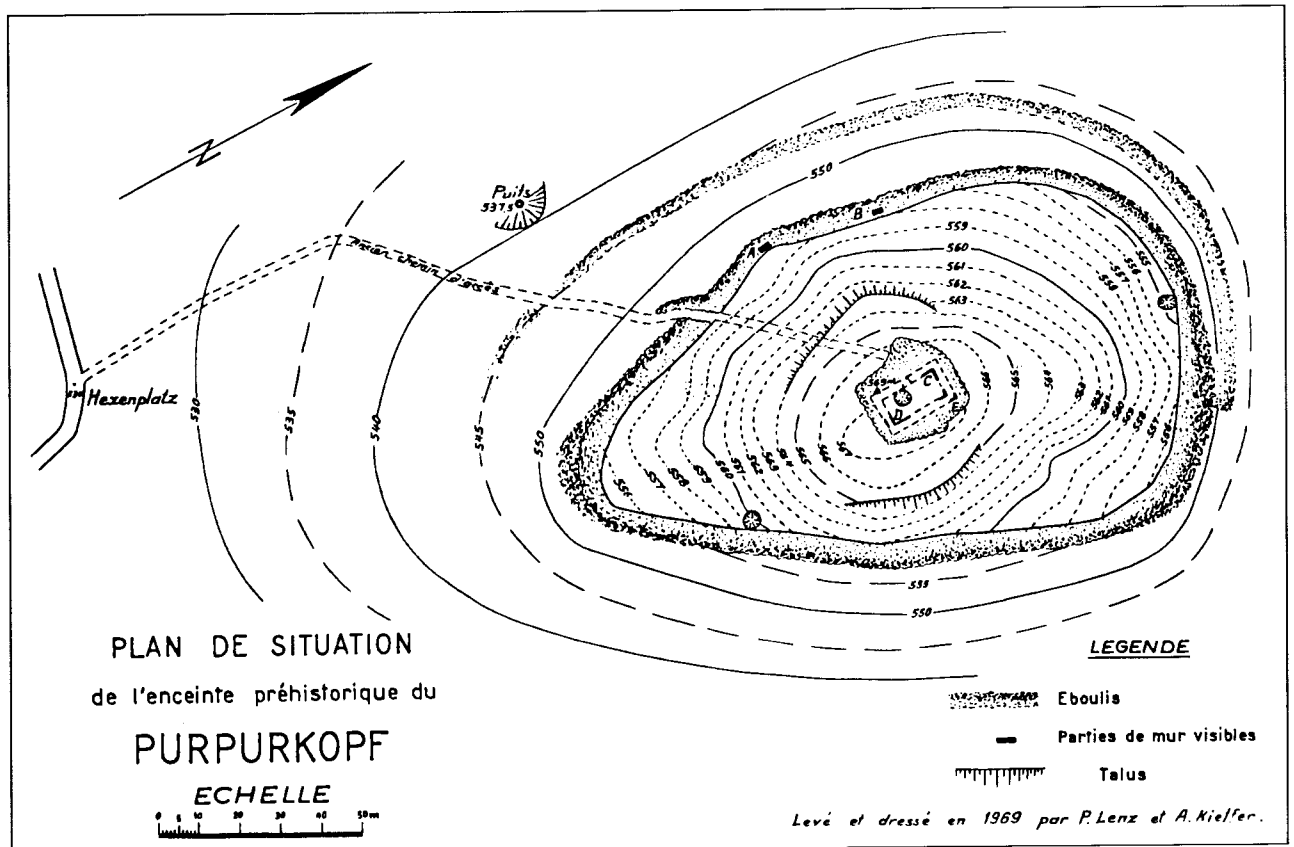
Abb. 3 Purpurkopf. Grundriß (Aufmaß Lenz/Kieffer 1969, in: CAAAH 1977).
