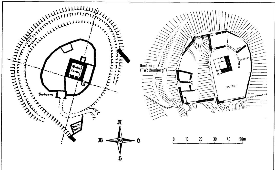
Abb. 16 Schlössel bei Klingenmünster (Pfalz) und Egisheim/Nord (F. Sprater in: Burgwart 39, 1938 und Th. Biller unter Verwendung des Grundrisses von H. Zumstein).
