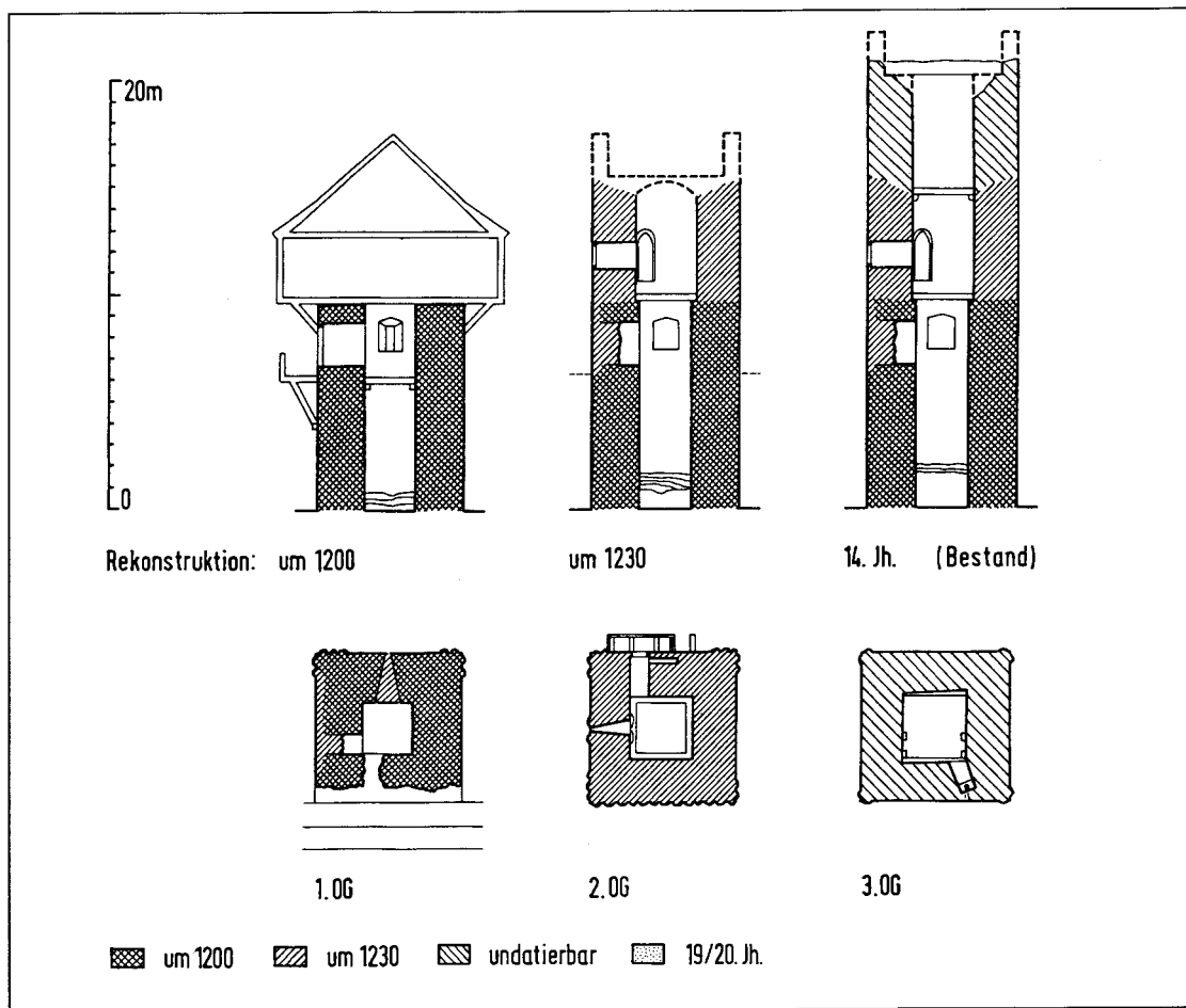
Abb. 15 Wineck. Entwicklung und Grundrisse des Turmes (Th. Biller).
