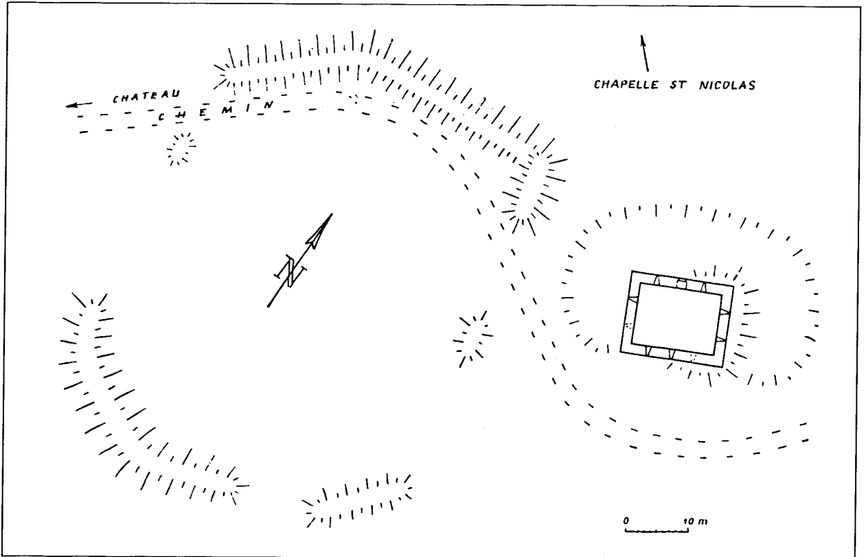
Abb. 12 Ottrott. Grundriß (H. Zumstein, in: CAAAH 15, 1971).
