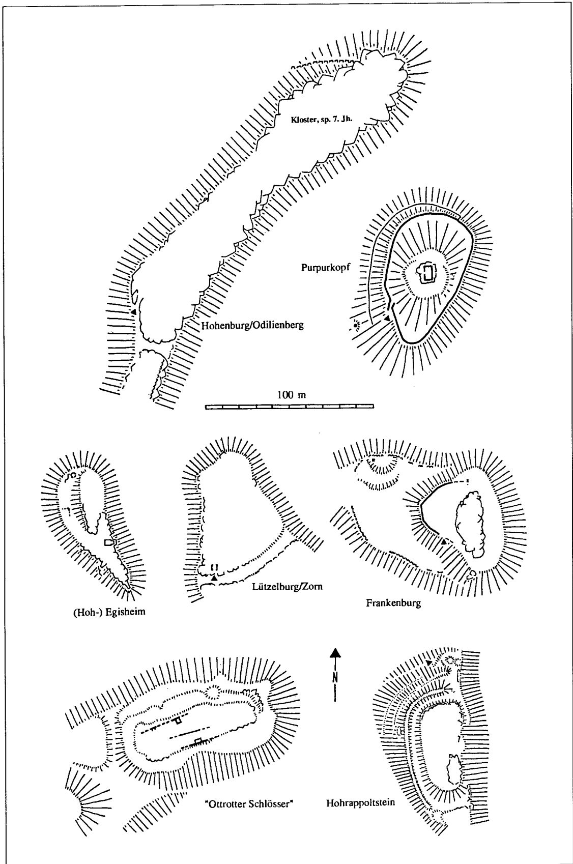
Abb. 2 Gräflische und andere große Burgen des 10.–12. Jhs. Die Abbildung dient vor allem der Darstellung der Gesamtanlagen und dem Größenvergleich. Alle Anlagen mit Ausnahme des Purpurkopfes sind später neu gestaltet worden; diese jüngeren Bauten, Gräben usw. hier weggelassen (Th. Biller).
