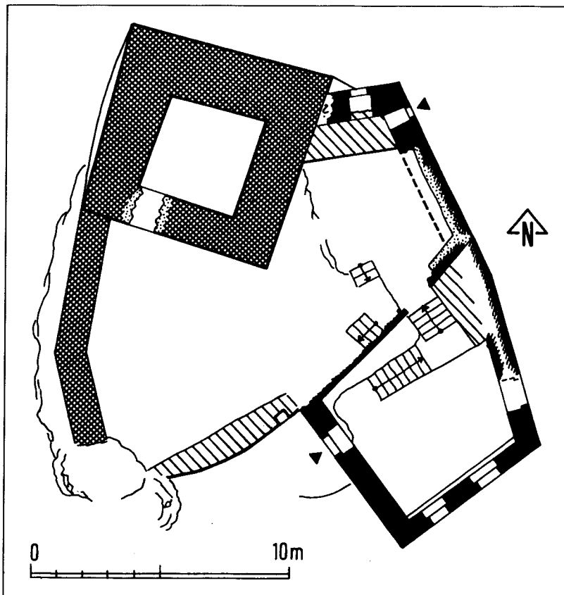
Abb. 17 St. Ulrich über Rappoltsweiler. Baualterplan der ältesten Teile (Wohnbau, Turm) auf dem nördlichen Felskopf (schwarz, kreuzschraffiert: Phasen des 12. Jhs., schraffiert: spätmittelalterlich) (Th. Biller unter Verwendung des Grundrisses von B. Ebhardt).
