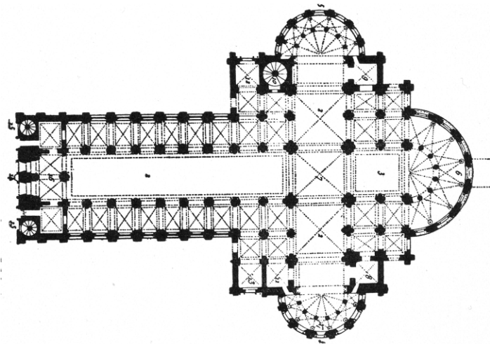
Abb. 171a) Tournai / Kathedrale, Grundriss um 1200
