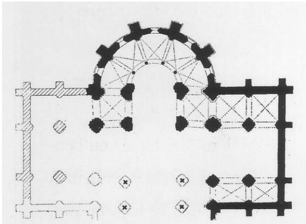
Abb. 153b) Roskilde, ursprünglicher Grundriss um 1170
