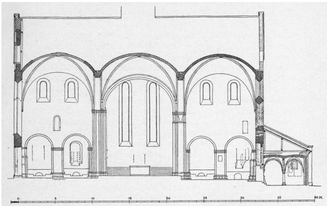
Abb. 73) Sorø, Ostwand
