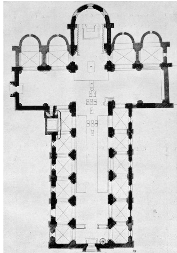
Abb. 20) Ringsted / St. Bendt, Grundriss
