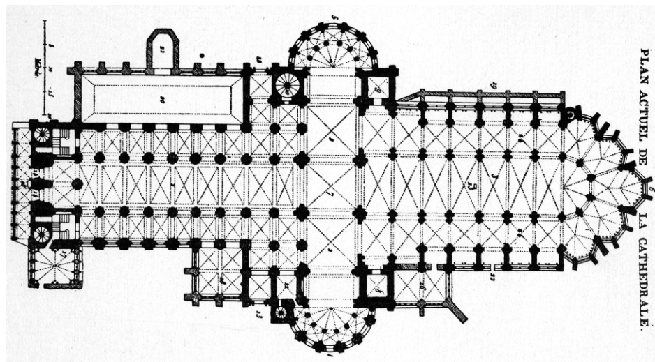
Abb. 171b) Tournai / Kathedrale, Grundriss (heutiger Zustand)
