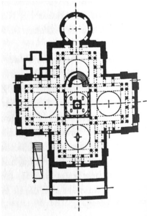
Abb. 122) Konstantinopel / Apostelkirche (ab 536), rekonstr. Grundriss
