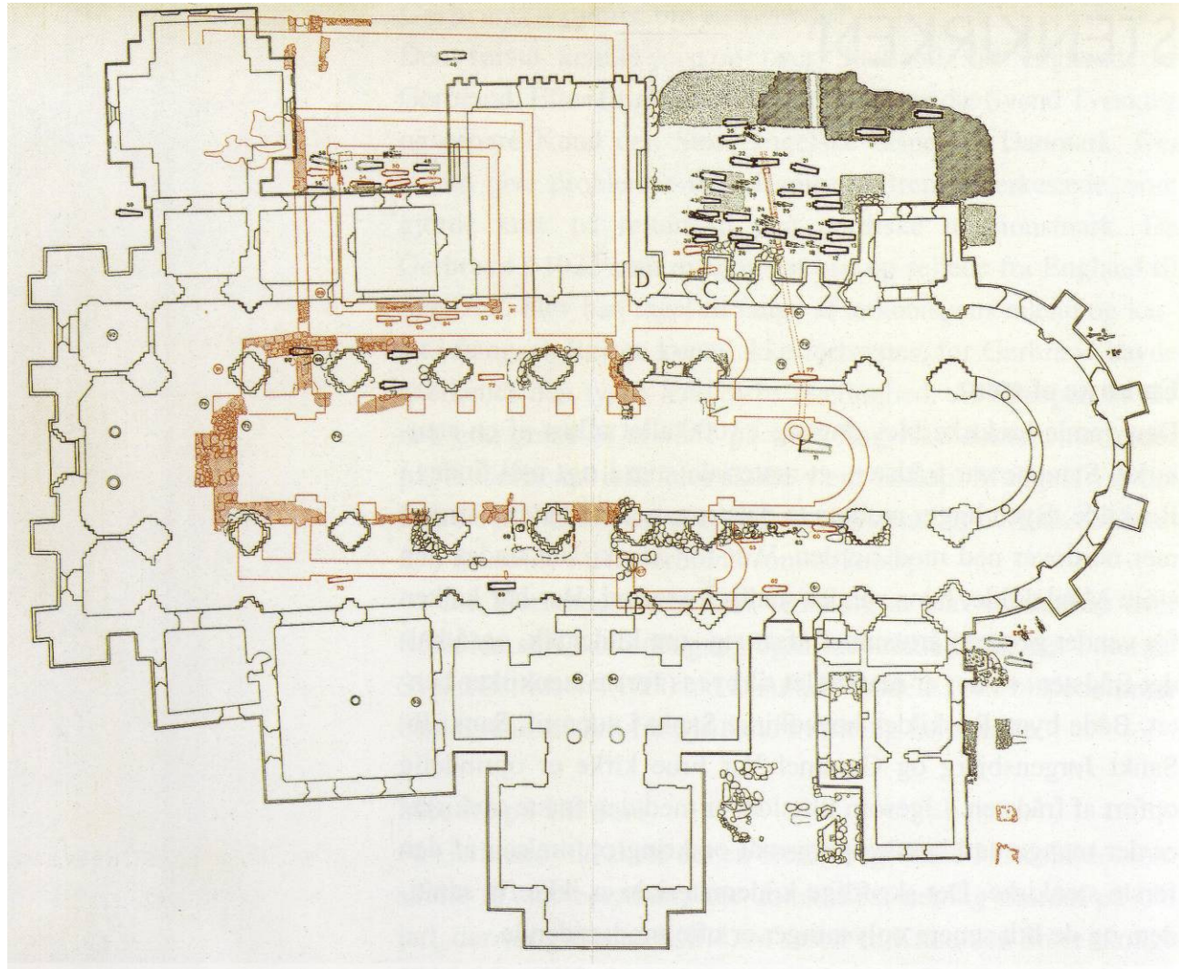
Abb. 152) Roskilde / Dom, Grundriss der heutigen Kirche (in Braun der Grundriss von Sven Estridsens Domkirche)
