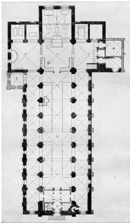
Abb. 50) Sorø, Grundriss
