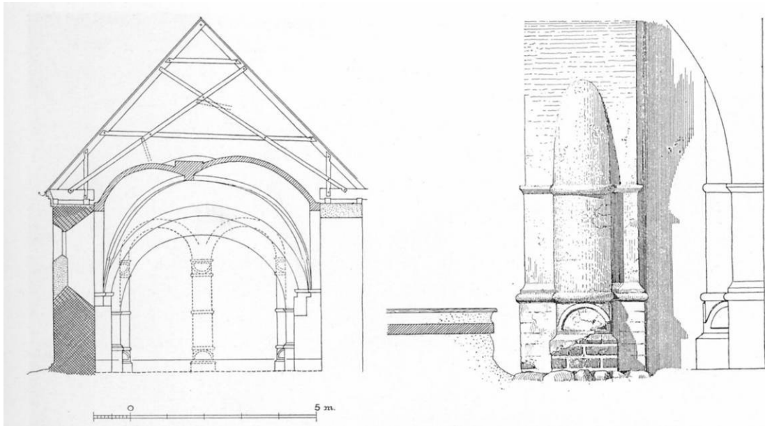
Abb. 119) Torup, Schnitt durch das Langhaus nach Westen (um 1200), Mittelsäule der Arkade von C. G. Schultz 1936 rekonstruiert
