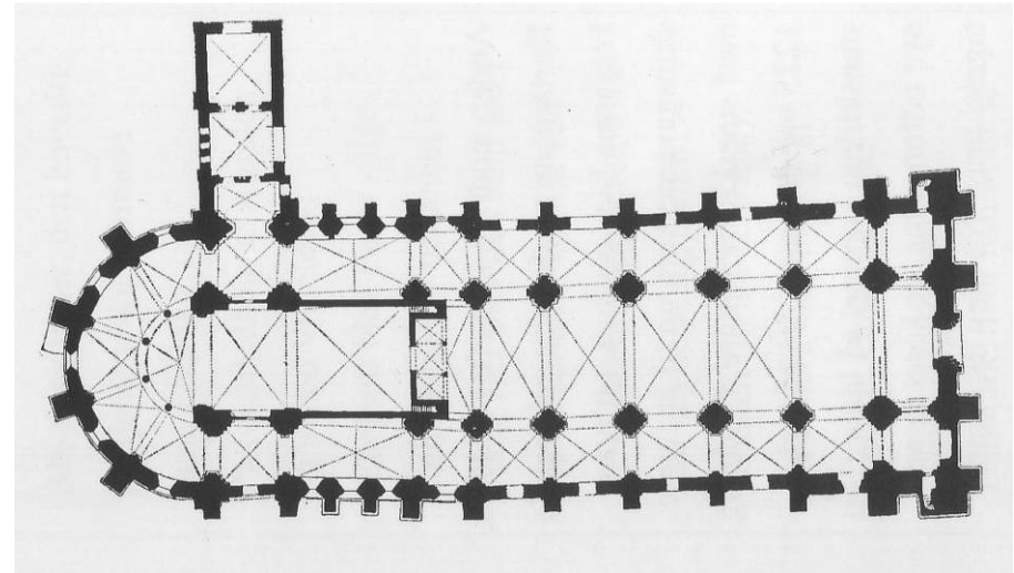
Abb. 132) Roskilde / Dom, Grundriss um 1280
