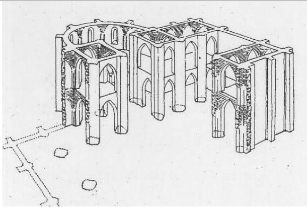
Abb. 153a) Roskilde, ursprünglicher Bauplan um 1170
