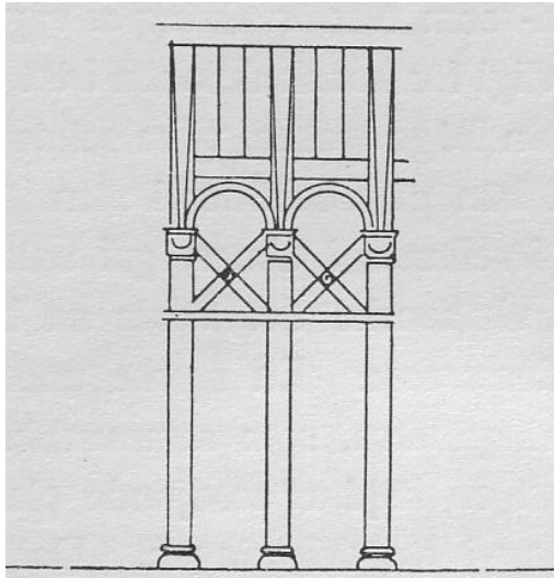
Abb. 126) Hopperstad / Stabkirche, Säulen des Langhauses
