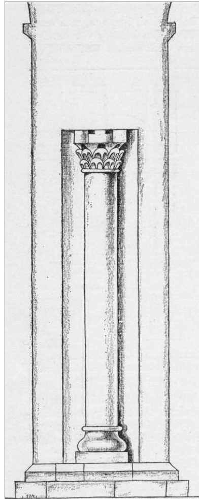
Abb. 182) Dalby, Nischensäule
