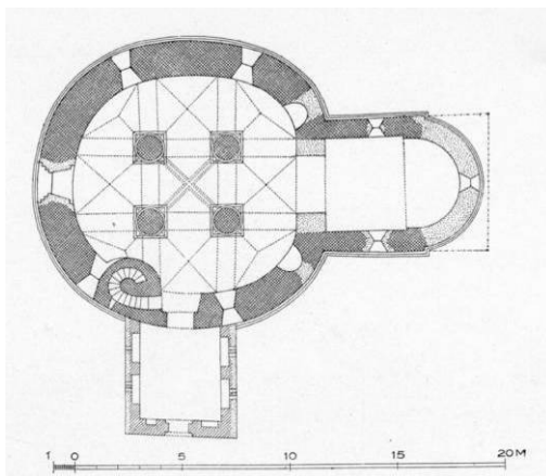
Abb. 87) Bjernede, Grundriss
