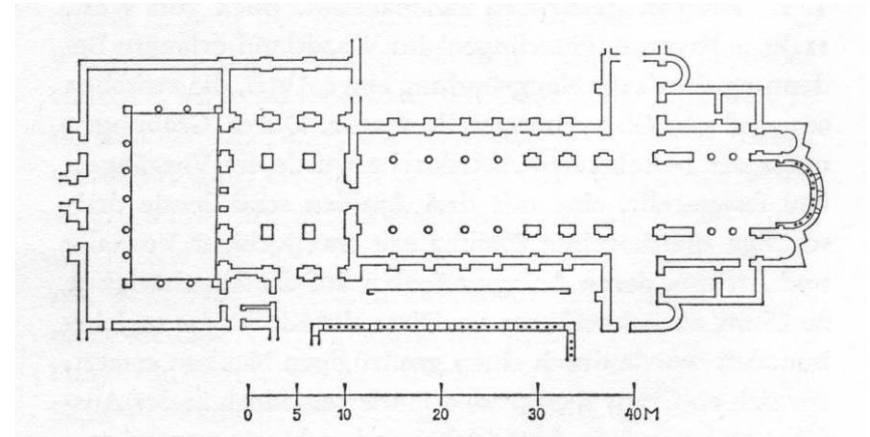
Abb. 47) Cluny II, Grundriss der ehemal. Abteikirche um 955 (Rekonstruktion)
