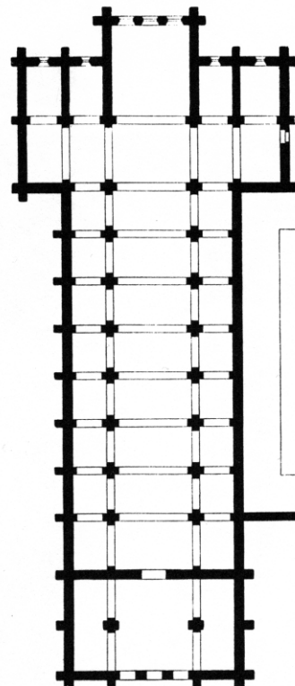
Abb. 51) Fontenay, Grundriss
