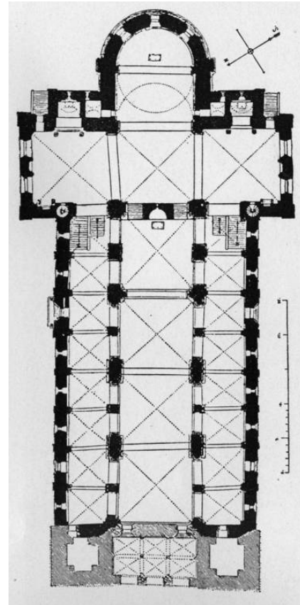
Abb. 15a) Lund / Dom, Rekonstruktion des ursprüngl. Grundrisses
