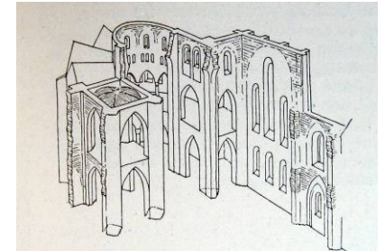
Abb. 158) Roskilde, 2. Planwechsel
