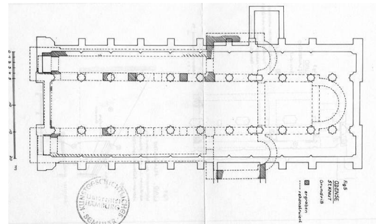
Abb. 48) Odense / St. Knud, heutige Kirche (mit Rekonstruktion des Vorgängerbaus)
