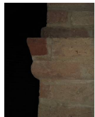
Abb. 93) Kämpferprofi
