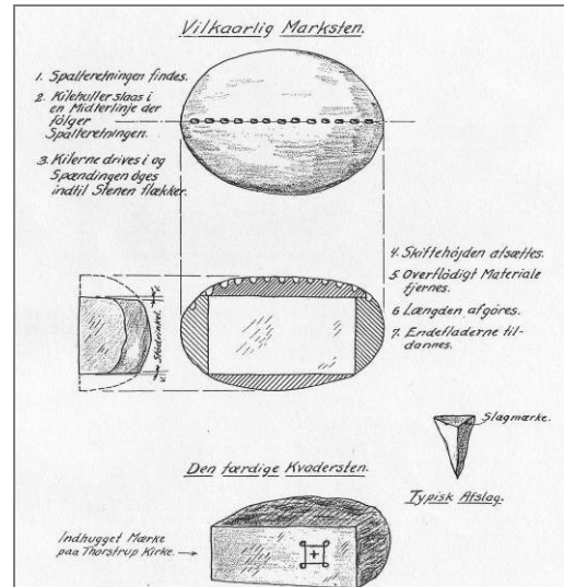
Abb. 193) Granitquaderherstellung: 1. Festle- gen der Spaltrichtung, 2. Einschlagen von Keil- löchern entlang der Spaltrichtung, 3. Eintreiben der Keile bis der Druck den Stein sprengt, 4.-7. Abarbeiten der restl. Flächen
