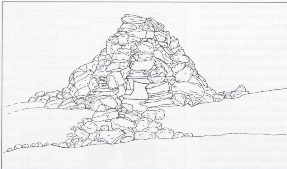
Abb. 2: Kuppelgrab ( dome grave ) KIR 005, Ansicht der Nordseite (Maßstab 1:40, Zeichnung J. Budka).
