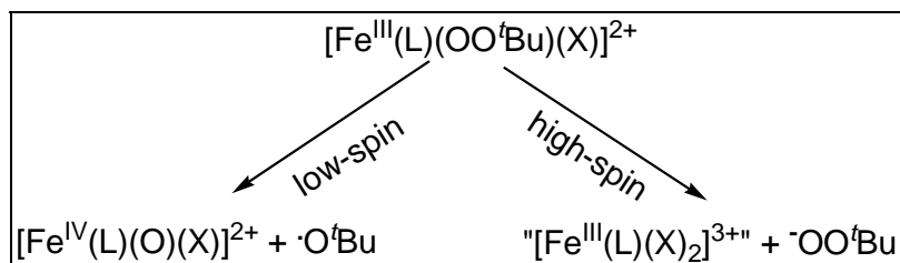
Formel 4-2: Zerfall einer Eisen(III)alkylperoxo-Verbindung
