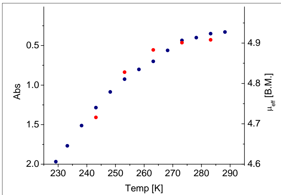
Abb. 2-5: Temperaturabhängigkeit des effektiven magnetischen Momentes und der Absorption bei 380 nm von [\text{Fe}(\text{L})(\text{OTf})_2] in MeCN in einem Bereich von +25 bis -40^\circ\text{C}
