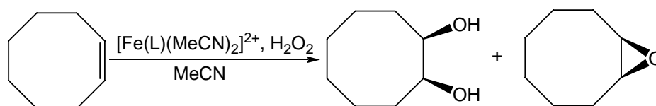
Abb. 3-2: Oxidation von Cycloocten mittels [\text{Fe}(\text{L})(\text{MeCN})_2]^{2+} und Wasserstoffperoxid
