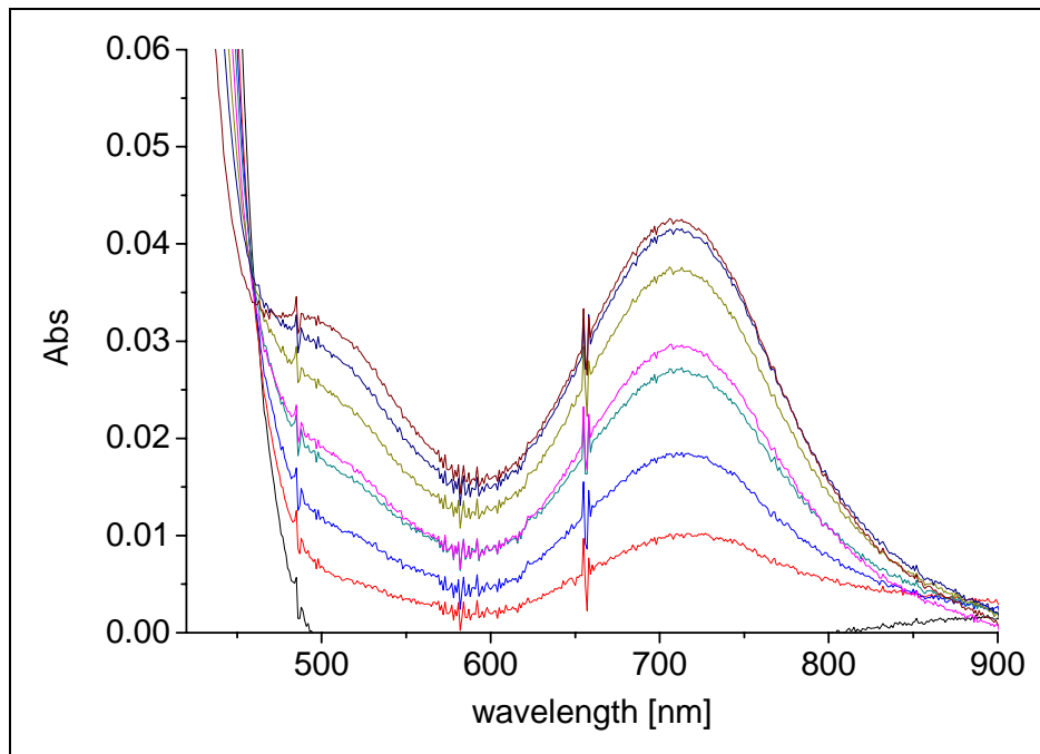
Abb. 5-15: Reaktion von [\text{Fe}(\text{L}_o)(\text{solv.})]^{2+} mit \text{H}_2\text{O}_2 in wässriger Lösung (0.05 M Citrat-Puffer, pH = 5.9, 0^\circ\text{C} ); Bildung der Bande innerhalb von 10 s
