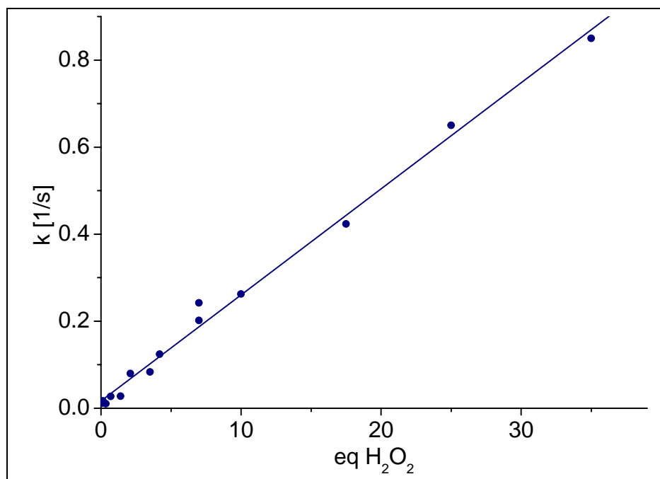
Abb. 5-4: Abhängigkeit der Geschwindigkeitskonstante von der H_2O_2 -Konzentration bei 0^\circ C in Wasser
