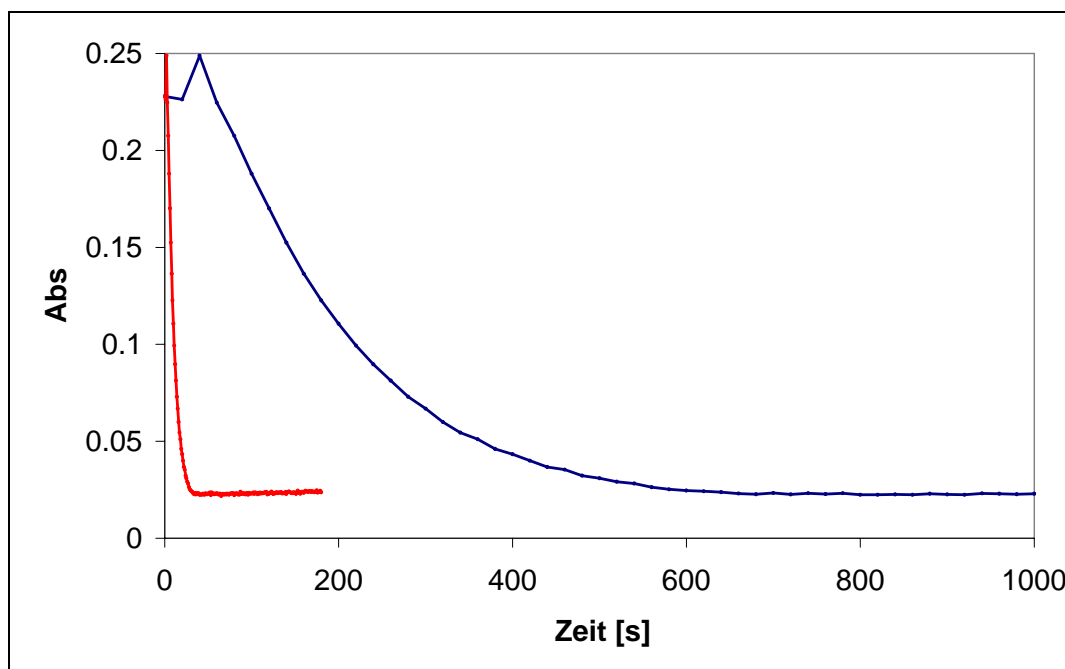
Abb. 5-6: Zerfall von [\text{Fe}^{\text{IV}}(\text{L}_n)(\text{O})]^{2+} bei Zugabe von \text{Fe}(\text{ClO}_4)_2 \cdot 6 \text{H}_2\text{O} bzw. [\text{Fe}(\text{L}_n)(\text{MeCN})(\text{BF}_4)_2 in neutralem Wasser bei 0^\circ\text{C}
