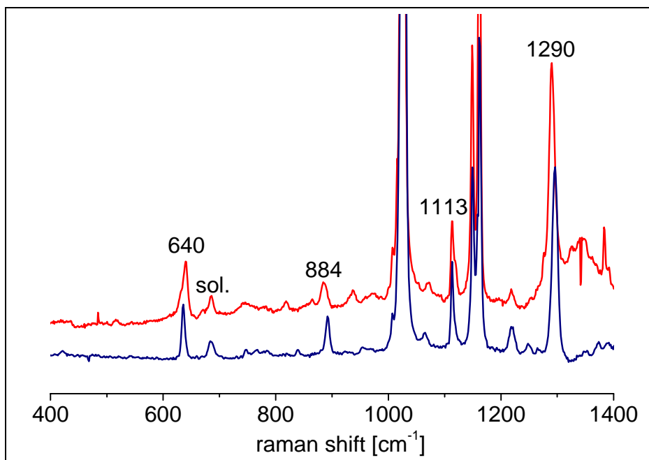
Abb. 4-5: Resonanz-Raman-Spektrum von Eduktkomplex (Blau, 413 nm Laser) und Intermediat (Rot, 453 nm Laser) der Reaktion von [\text{Fe}(\text{L})(\text{OTf})] mit 2 \text{ eq } \text{KO}_2 in MeOH bei -40^\circ\text{C} ; aufgenommen bei 77 K
