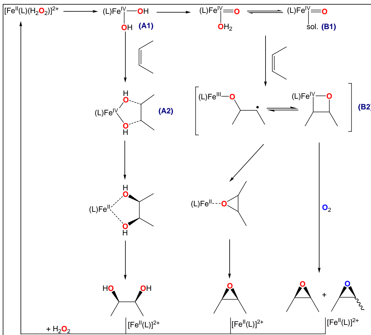
Abb. 6-1: Katalysezyklus der Oxidation von Olefinen mit [\text{Fe}(\text{L})]^{2+}
