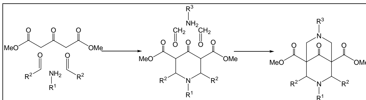
Abb. 2-2: Synthese von Bispidonliganden
