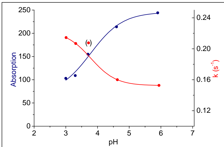
Abb. 5-9: Einfluss des pH-Werts auf Ausbeute und Geschwindigkeit in 0.05 M Acetatpuffer der Bildung von [Fe(L_n)(O)]^{2+} bei 0°C durch Reaktion mit 10 eq H_2O_2
