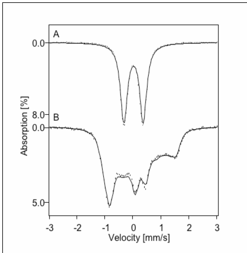
Abb. 5-3: 4.2K Mössbauer-Spektrum von Verbindung 2 aufgenommen mit B = 0 T (A) und B = 8.0 T (B). Die durchgezogenen Linien sind simulierte Spektren mit D = +23(2) \text{ cm}^{-1} , E/D = 0 (fest), g = 2.0 , A_x/g_n\beta_n = -22(2) \text{ T} , A_y/g_n\beta_n = -22(2) \text{ T} , A_z/g_n\beta_n \sim -5 \text{ T} , \Delta E_Q = 0.69(1) \text{ mm/s} , \eta = 0.5 , \delta = 0.02 \text{ mm/s} (relativ zu Eisen bei 298 K) and \Gamma = 0.29 \text{ mm/s} .
