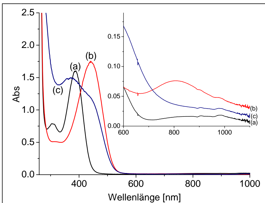
Abb. 4-2: UV-vis-Spektrum des Intermediates der Reaktion von [\text{Fe}(\text{L})(\text{OTf})_2] und 2\text{eq KO}_2 in Methanol bei -40^\circ\text{C} ; schwarz: Eduktspektrum (a); rot: Intermediatspektrum, nach 5 Minuten (b) blau: Zerfallsspektrum, nach 60 Minuten, bei -20^\circ\text{C} (c)
