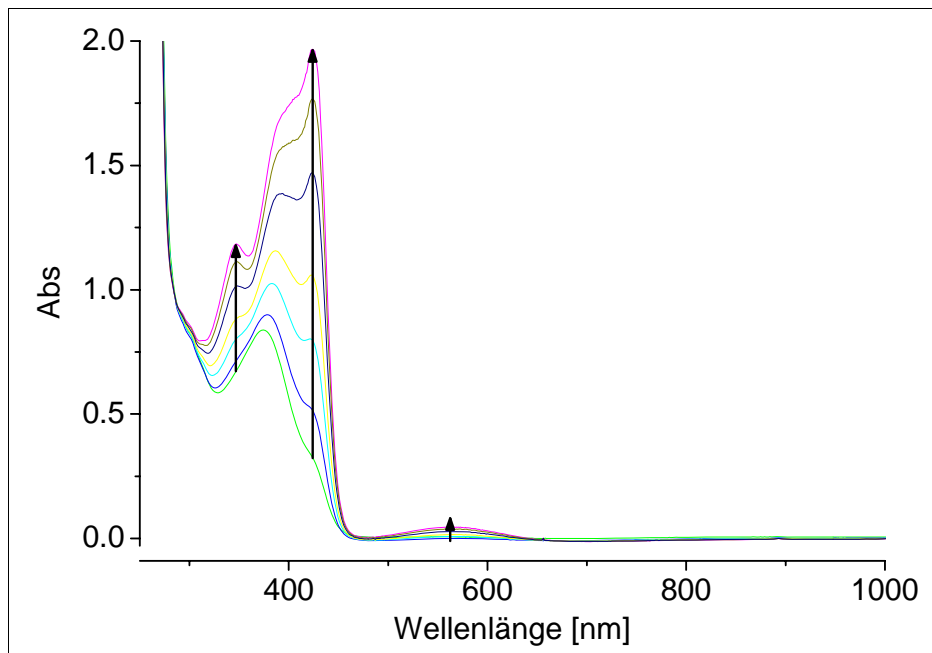
Abb. 2-4: Temperaturabhängigkeit des optischen Spektrums von [Fe(L)(OTf) 2 ] in MeCN beim Abkühlen von +25°C auf -44°C
