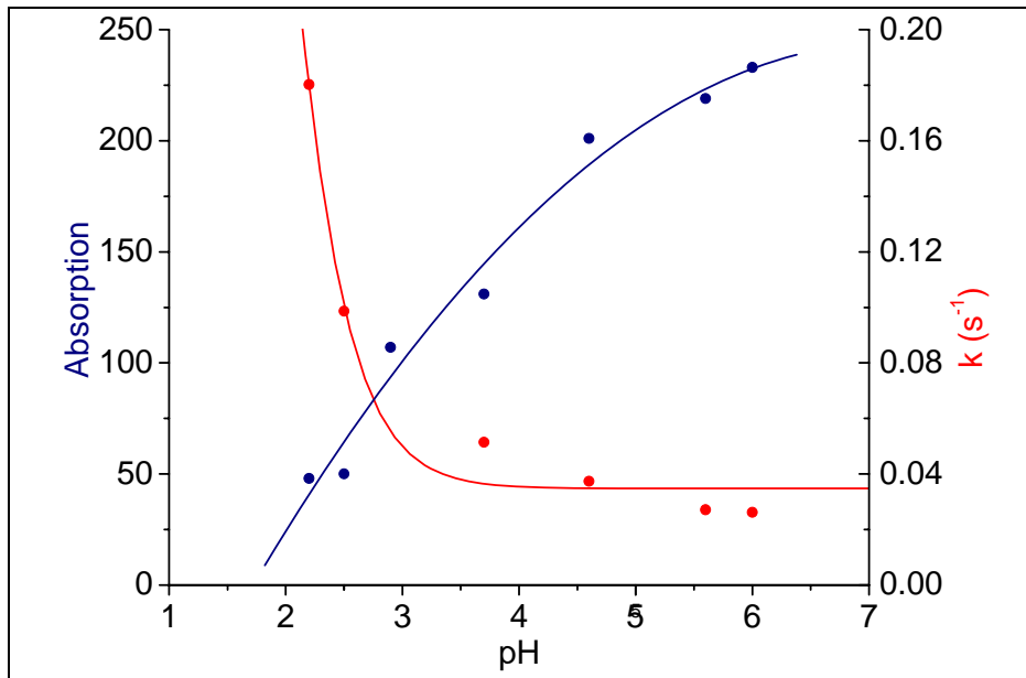
Abb. 5-8: Einfluss des pH-Werts auf Ausbeute und Geschwindigkeit in 0.05 M Citratpuffer der Bildung von [Fe(L_n)(O)]^{2+} bei 0°C durch Reaktion mit 10 eq H_2O_2
