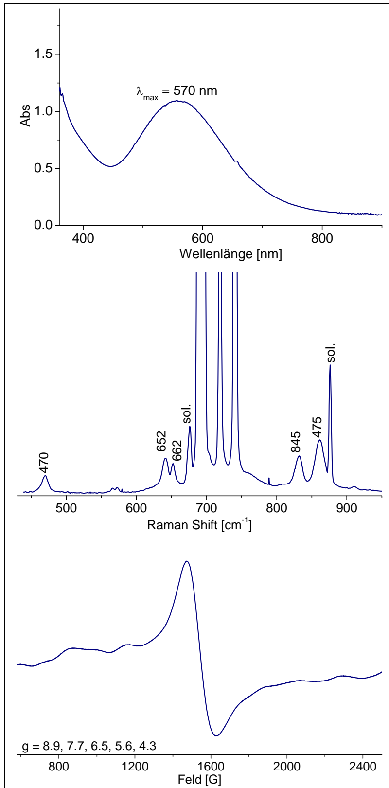
Abb. 4-10: Spektren des Alkylperoxy-Komplexes [\text{Fe}(\text{L})(\text{OO}^t\text{Bu})(\text{X})]^{2+} in \text{CH}_2\text{Cl}_2 oben: UVvis bei 233 K; Mitte: Resonanz-Raman bei 77 K (aufgenommen mit einem 568 nm Laser); unten: ESR bei 130 K
