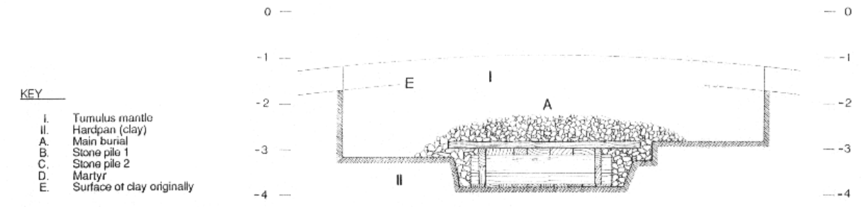
Abb.1 Tumulus G, Holzkammer, W-O Schnitt
