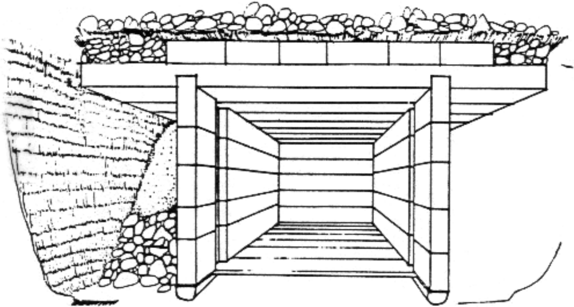
Abb.1 Tumulus B.T., Rekonstruktion der Holzkammer
