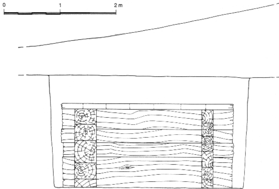
Abb.2 Tumulus N, Holzkammer, W-O Schnitt
