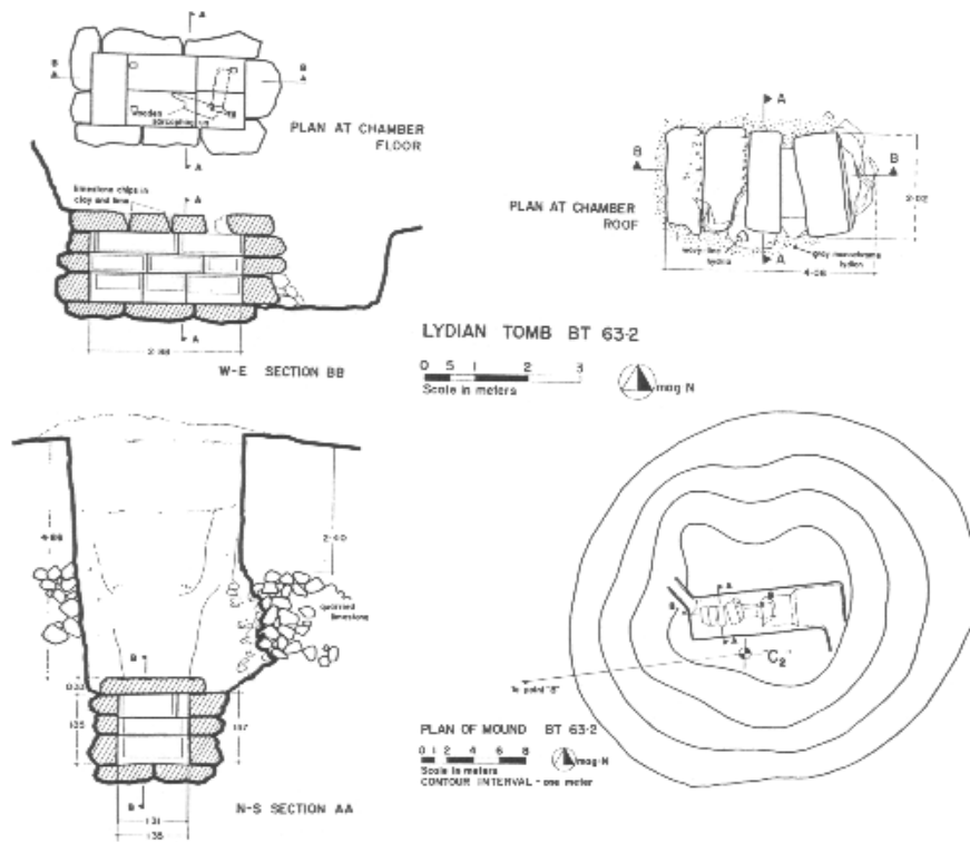
Abb.2 Tumulus BT 62 2, Grundriß und Schnitte
