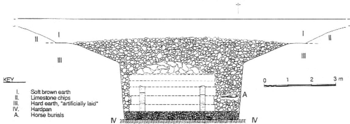
Abb.3 Tumulus KY, Holzkammer, W-O Schnitt
