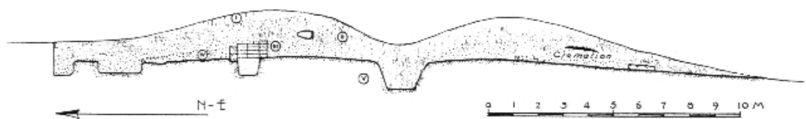
Abb.2 Tumulus F, Schnitt
