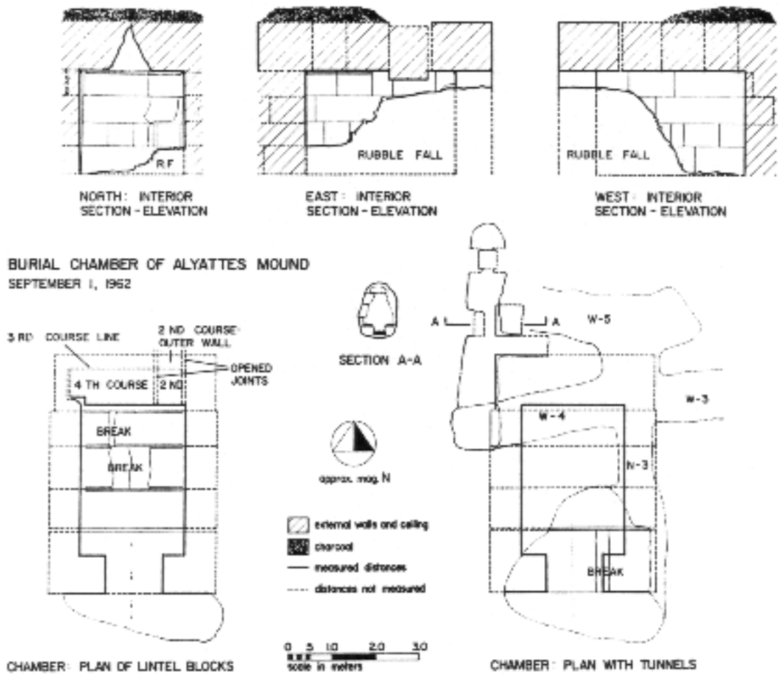
Abb.1 Alyattesgrab, Schnitte und Grundriß der Grabkammer
