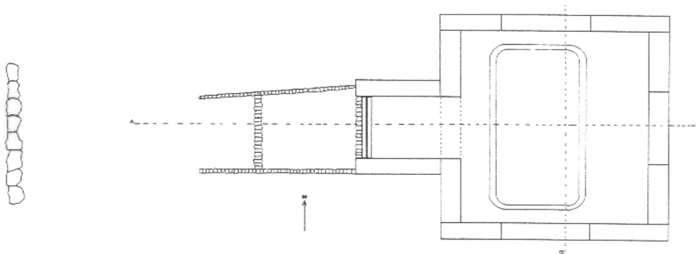
Abb.2 Basmacitepe, Plan der Grabanlage
