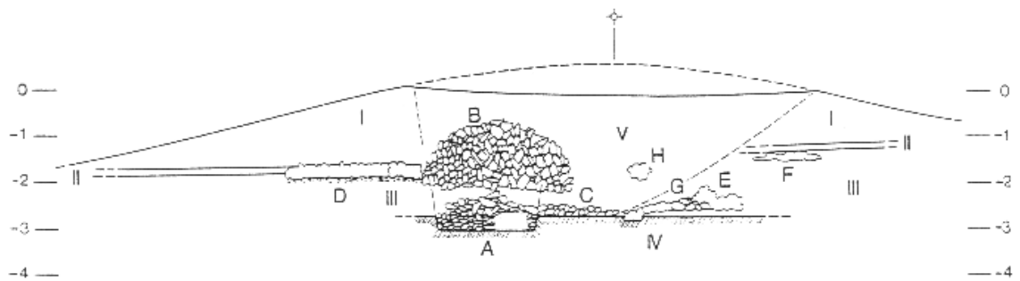
Abb.3 Tumulus C, Kammergrab, W-O Schnitt
