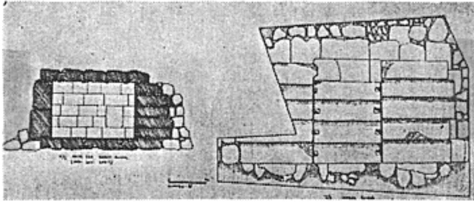
Abb.1 Tumulus T 1 Alahidir, Grabkammer, Längsschnitt und Aufsicht
