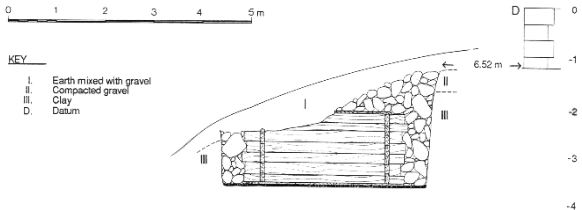
Abb.2 Tumulus J, Holzkammer, Schnitt
