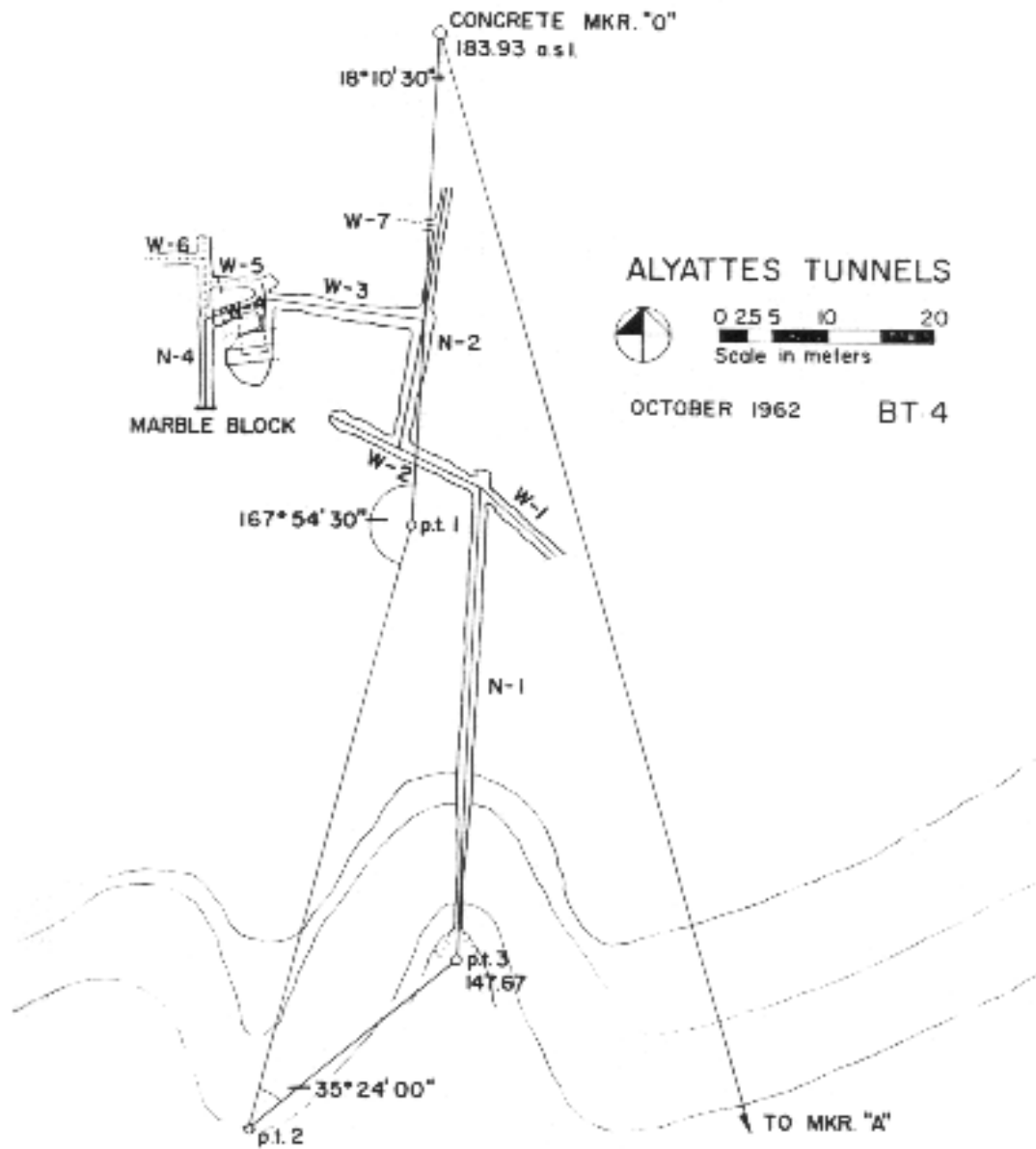
Abb.1 Alyattesgrab, Plan der Suchtunnel
