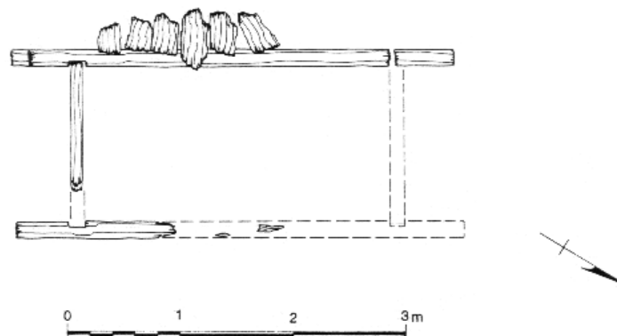
Abb.3 Tumulus Y, Holzkammer
