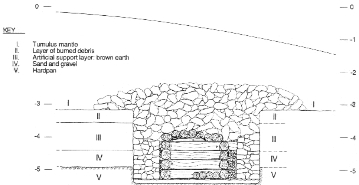
Abb.2 Tumulus N, Holzammer, N-S Schnitt
