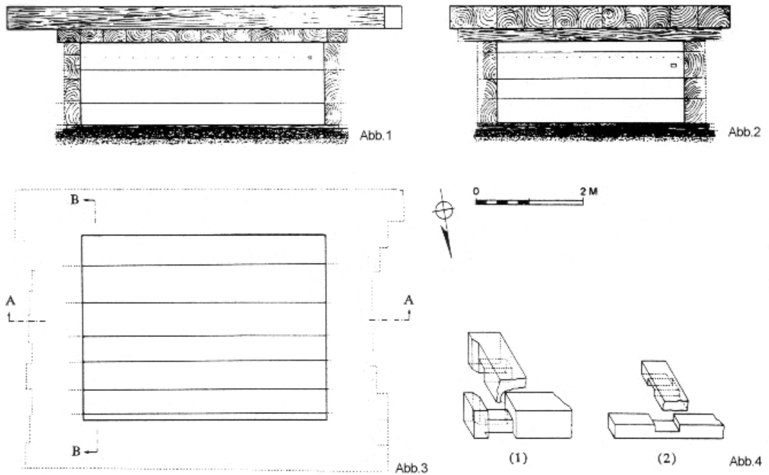
Abb.1 Tumulus P, Holzkammer, W-O Schnitt
