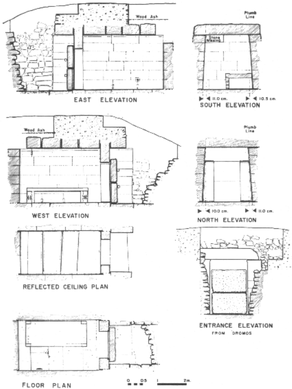
Abb.1 Tumulus BK 71, 1 Grabkammer, Plan und Schnitte
