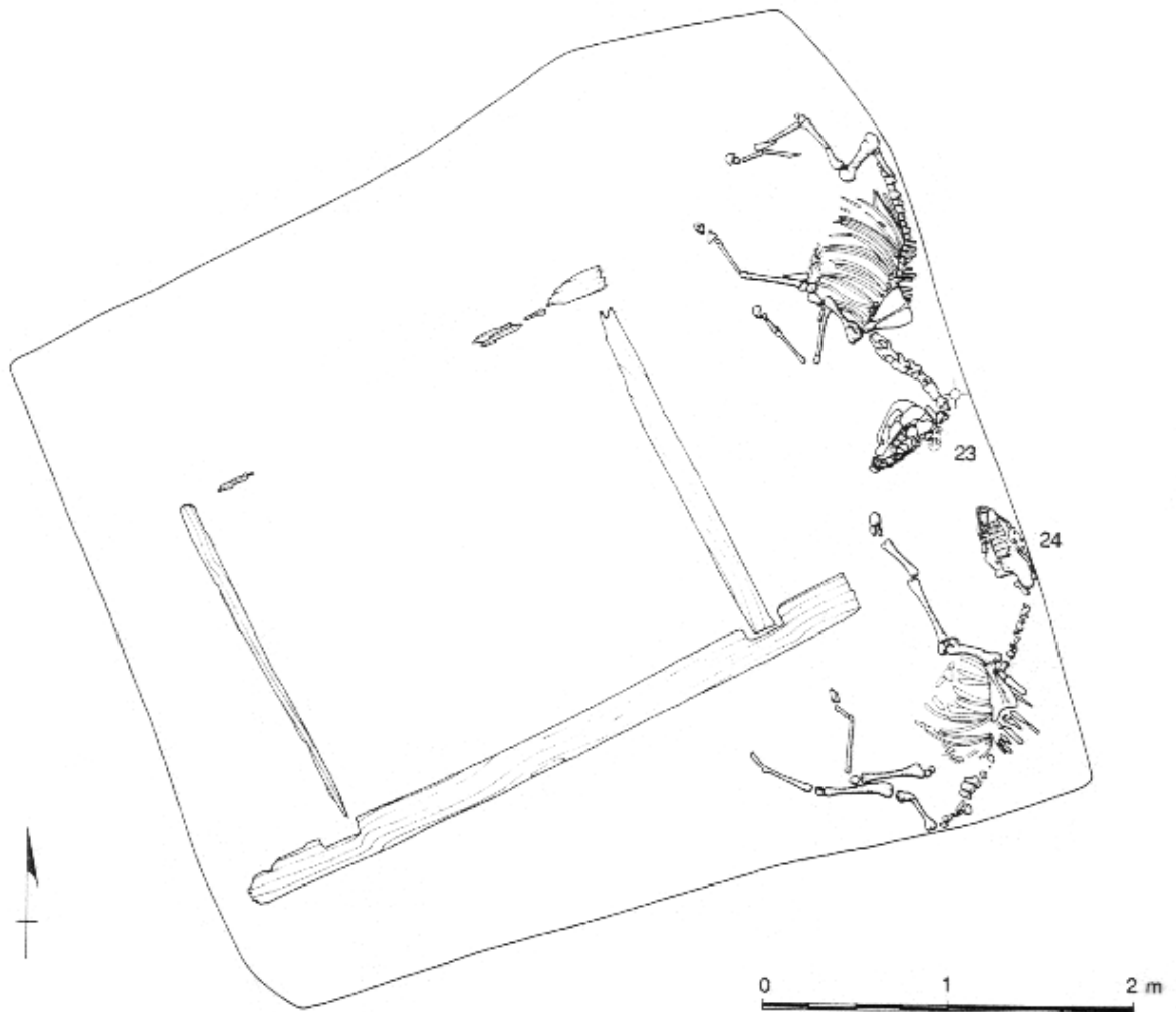
Abb.1 Tumulus KY, Holzkammer und Grube
