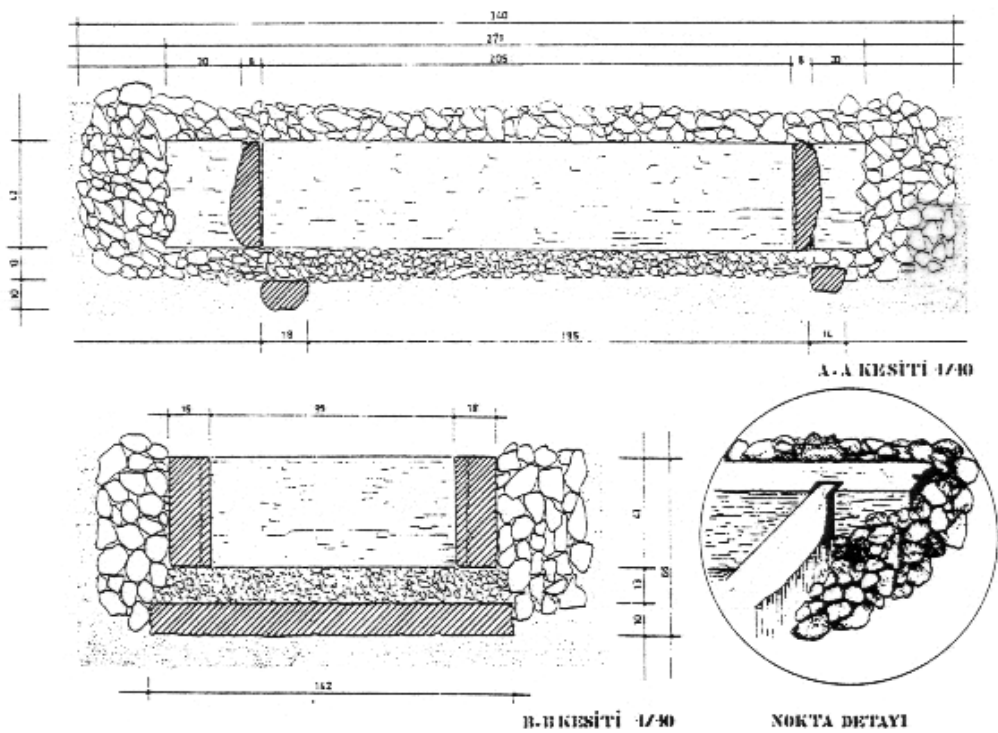
Abb.2 Kizlarkayasi, Schnitte und Detail der Holzkonstruktion in Tumulus A
