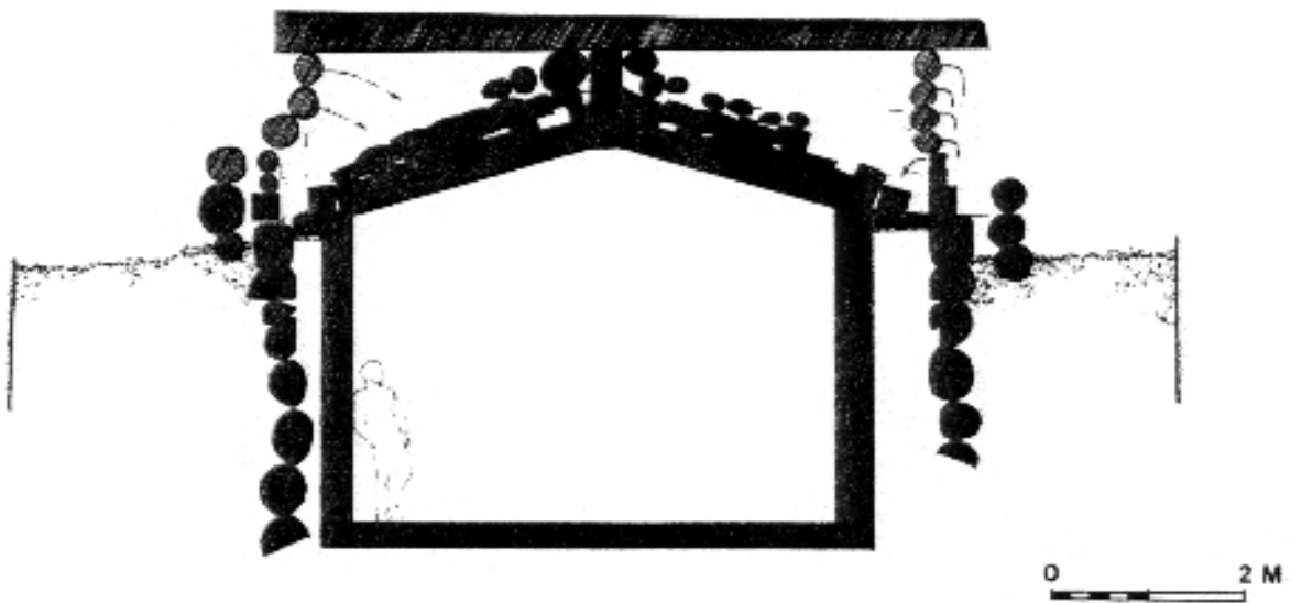
Abb.2 Tumulus MM, Holzkammer, W-O Schnitt
