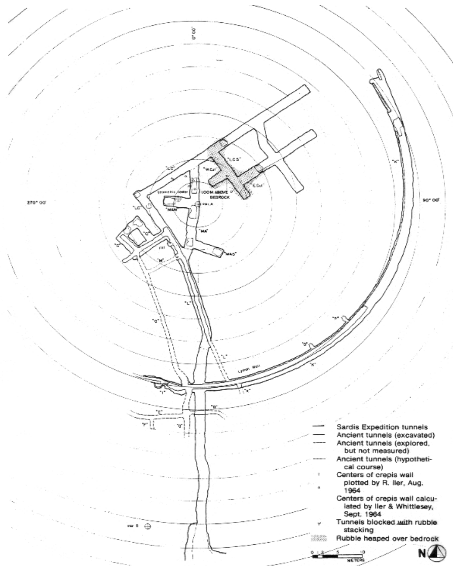
Abb.2 Karniyariktepe, Plan der Suchtunnel und der Krepismauer
