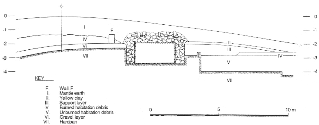
Abb.3 Tumulus H, Holzkammer, N-S Schnitt
