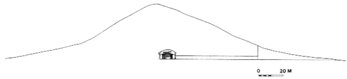
Abb.2 Tumulus MM, Schnitt
