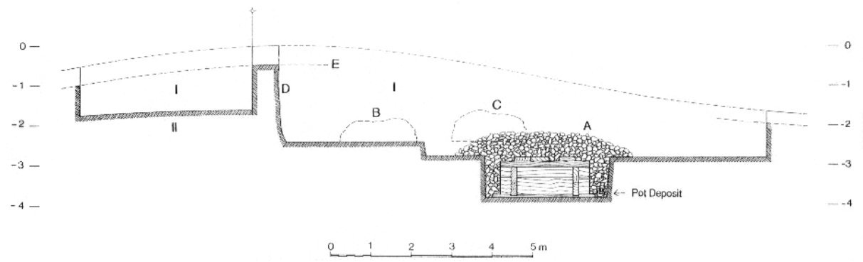
Abb.2 Tumulus G, Holzkammer, N-S Schnitt
