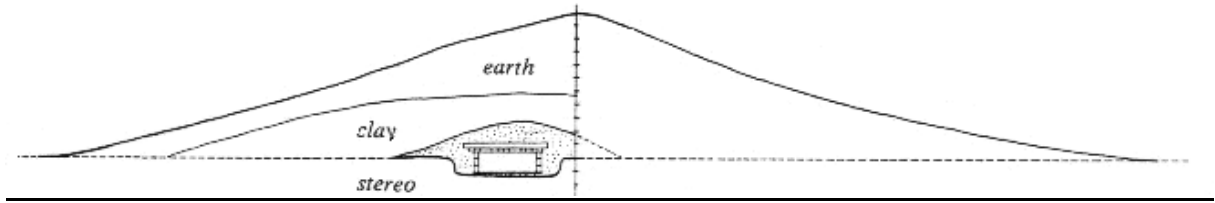
Abb.1 Tumulus P, Schnitt
