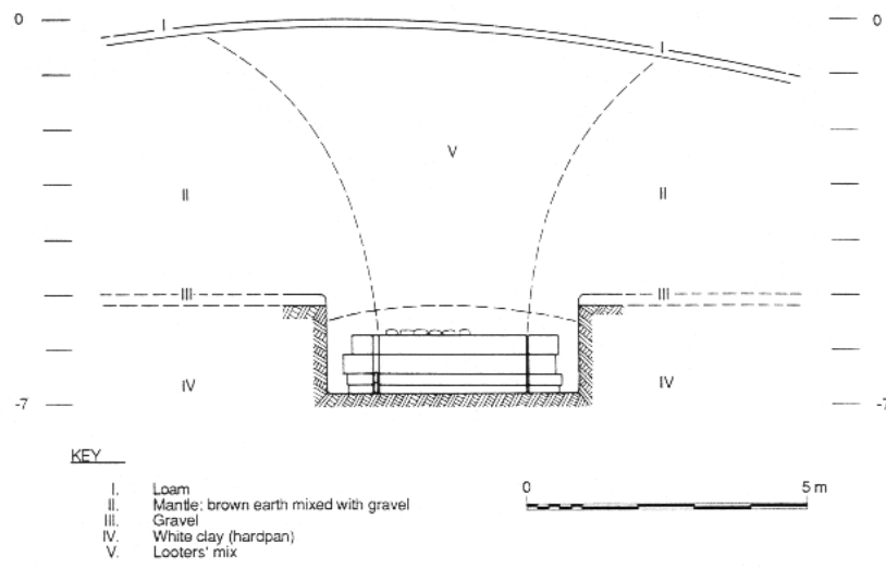
Abb.2 Tumulus Y, Holzkammer, N-S Schnitt
