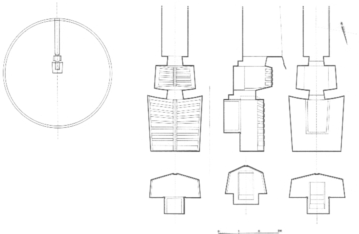
Abb.1 Tumulus A1, Grundriß und Details der Grabanlage
