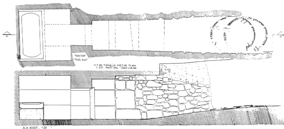
Abb.3 Tumulus BT 89, Grabkammer und Dromos, Plan und Längsschnitt
