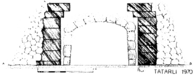
Abb.2 Tatarli, Schnitt durch die Grabkammer
