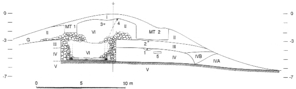
Abb.1 Tumulus S1, Holzkammer, N-S Schnitt
