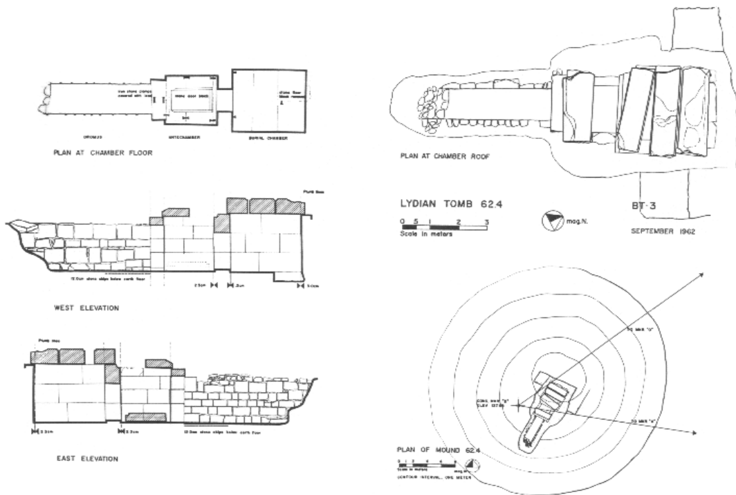
Abb.1 Tumulus BT 62.4, Grundriß und Schnitte
