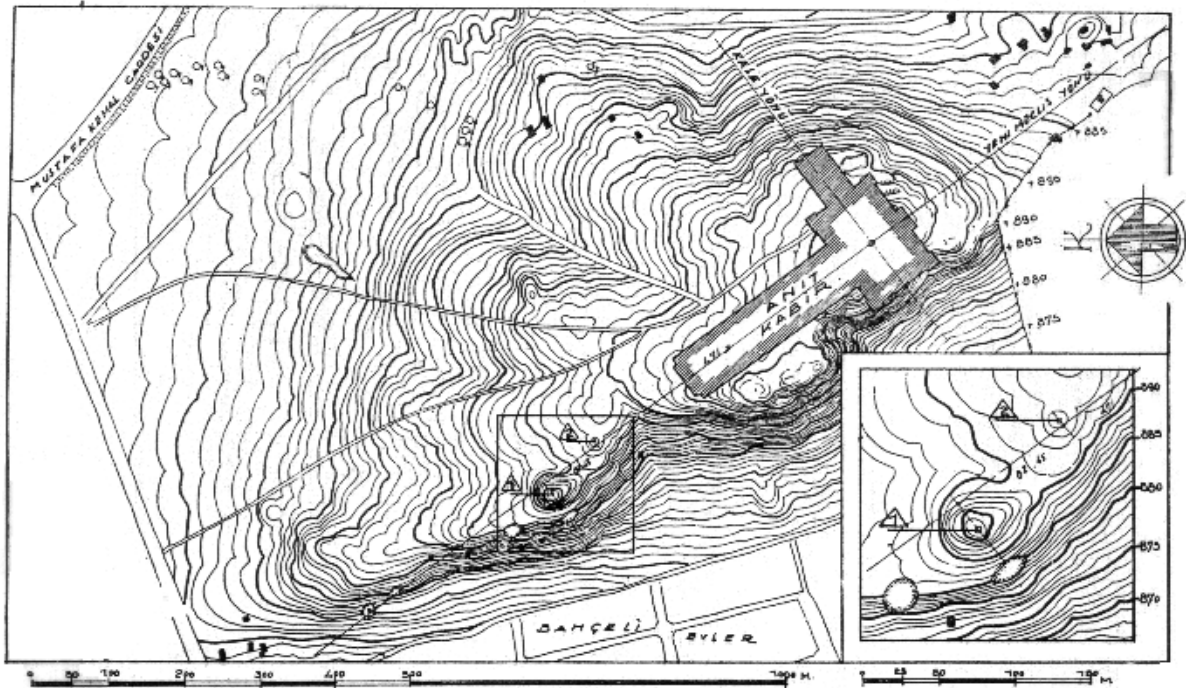
Abb.1 Plan des Anıttepe
