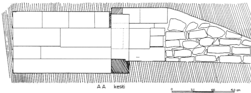
Abb.3 Basmacitepe, Schnitt der Grabanlage
