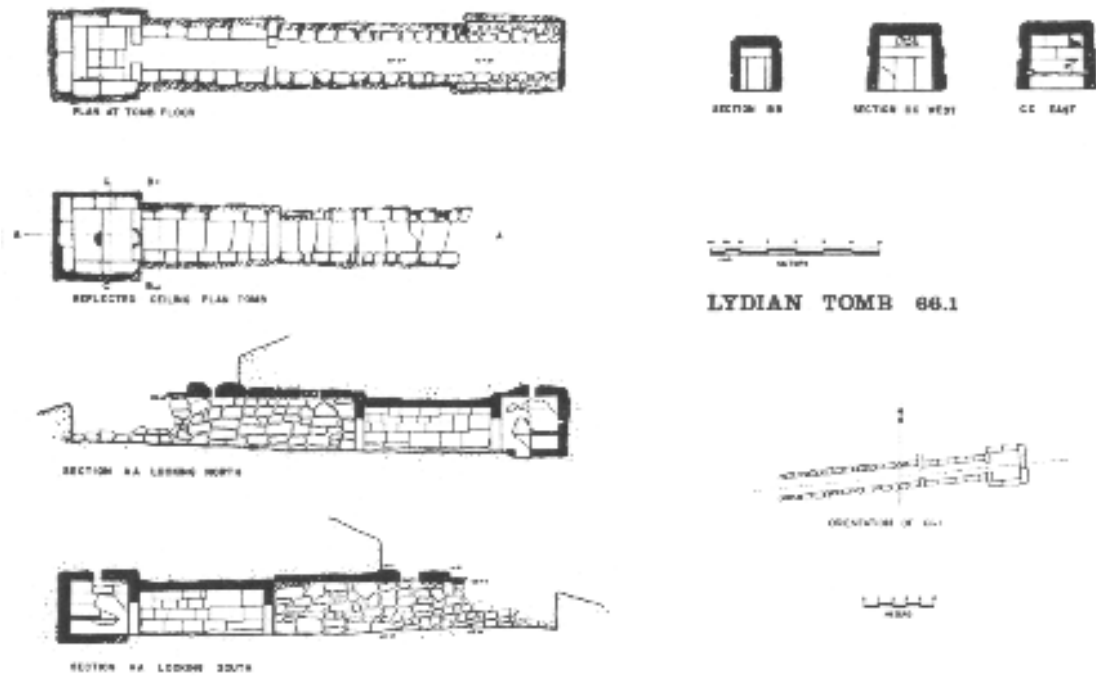
Abb.1 Tumulus BT 66.1, Grundriß und Schnitte der Grabkammer
