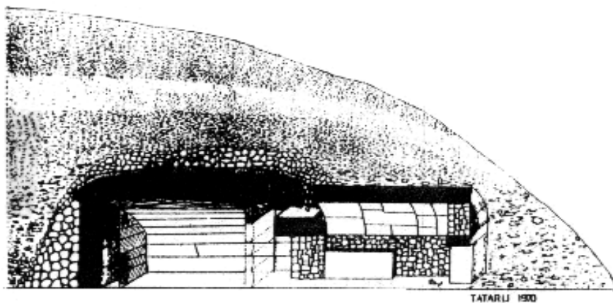
Abb.3 Tatarli, isometrischer Aufriß der Grabkammer
