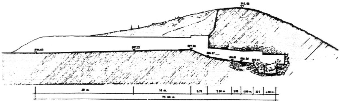
Abb.2 Tumulus B.T., Schnitt
