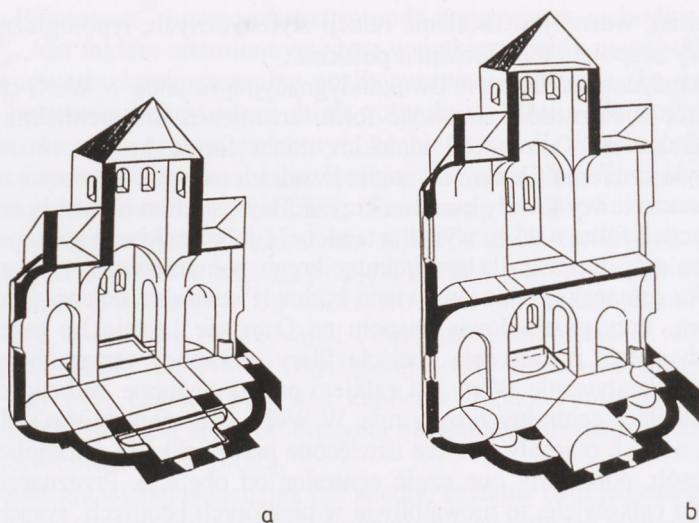
II. 7. Ostrów Lednicki, baptysterium – kaplica pałacowa, przekrój perspektywiczny, rekonstrukcja (wg Węclawowicz, Rosół). a) Faza I. b) Faza II
