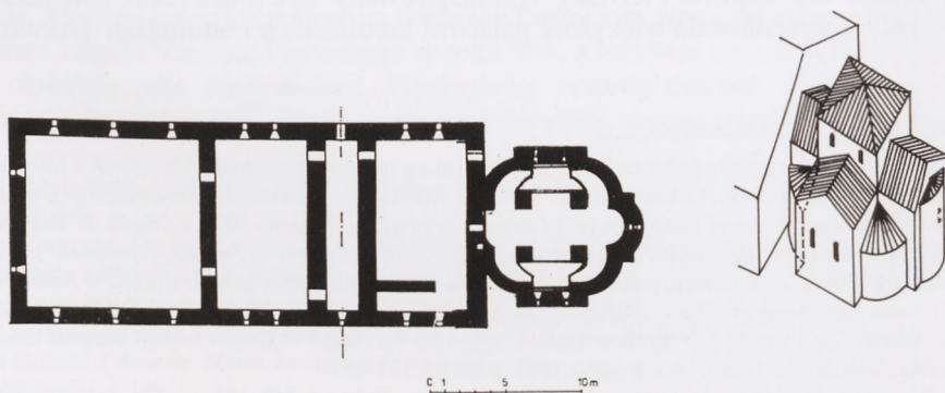
II. 9. Ostrów Lednicki, baptysterium – kaplica pałacowa, rzut poziomy i rekonstrukcja bryły, faza I (wg Rosół)
