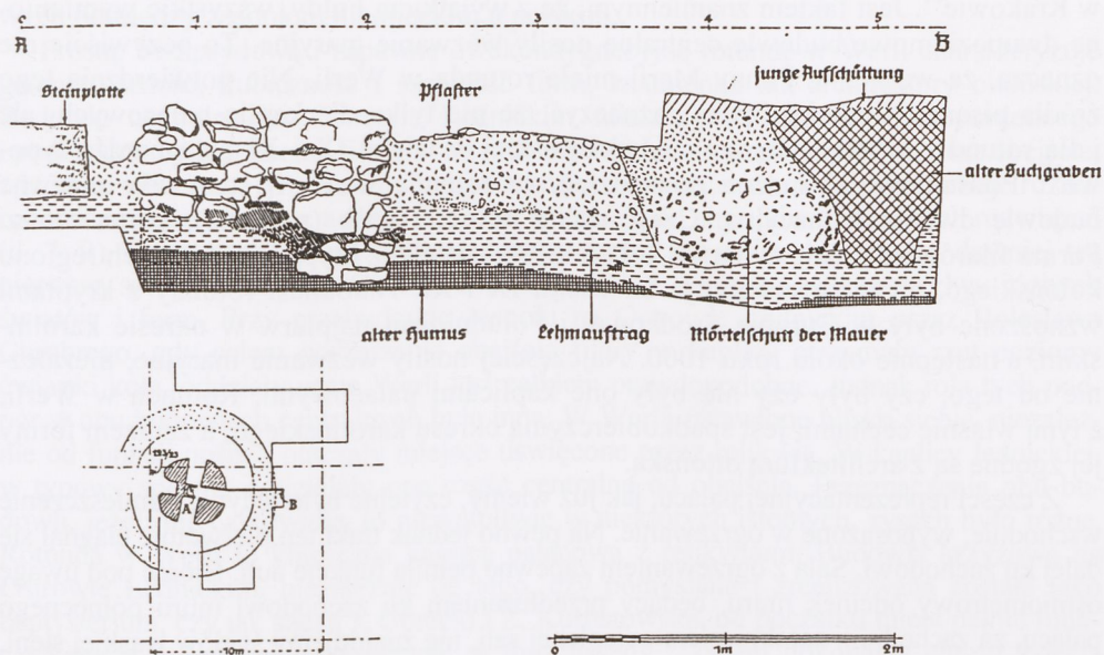
Il. 5. Werla, rotunda, przekrój na osi wschód-zachód (wg Schroller)
