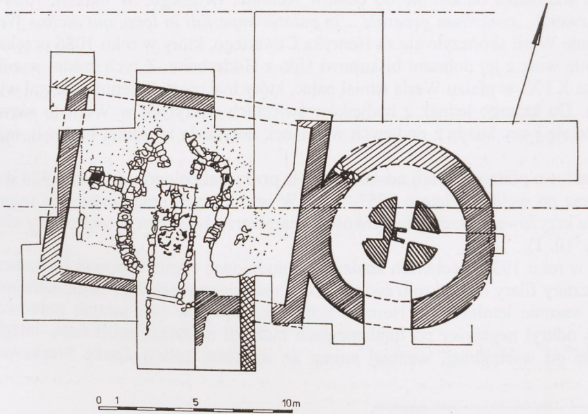
II. 2. Werla, rzut poziomy pałacu i rotundy (wg Schroller)
