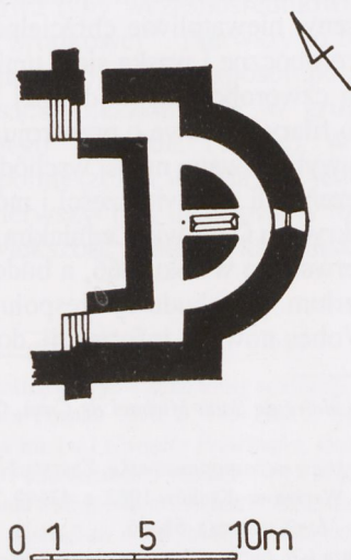
Il. 6. Kolonia, kościół Świętego Pantaleona, rzut poziomy krypty wschodniej z w. X (wg Kubach, Verbeek)
