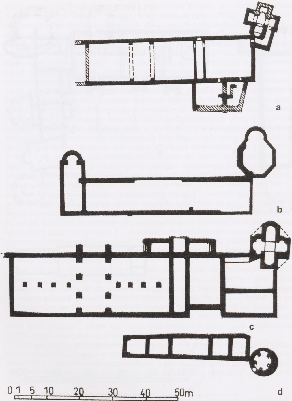
II. 12. Wczesnośredniowieczne pałace zespolone z kaplicą – typ drugi: a) Zürich, rzut poziomy pałacu ottońskiego (wg Binding); b) Bamberg, rzut poziomy pałacu biskupiego (wg Mayer); c) Goslar, rzut poziomy pałacu cesarskiego (wg Binding); d) Esztergom, rzut poziomy pałacu królewskiego (wg Żurowska)
