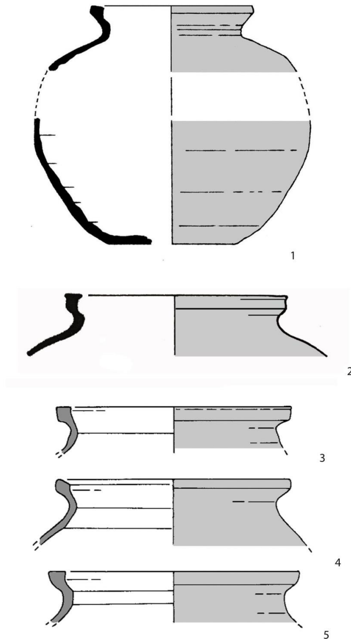
Textabb. 4: Fragmente der späten Älteren gelben Drehscheibenware (Typ Willigartaburg) aus Billigheim-Ingenheim (1), von Burg Anebos (2) und von der Willigartaburg (3-5). o.M.
