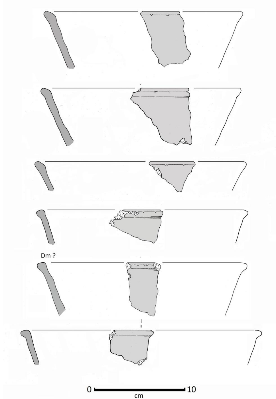
Textabb. 5: Schalen und Schüsseln der Älteren gelben Drehscheibenware aus dem zweiten Töpferofen in Wiesloch (1995)
