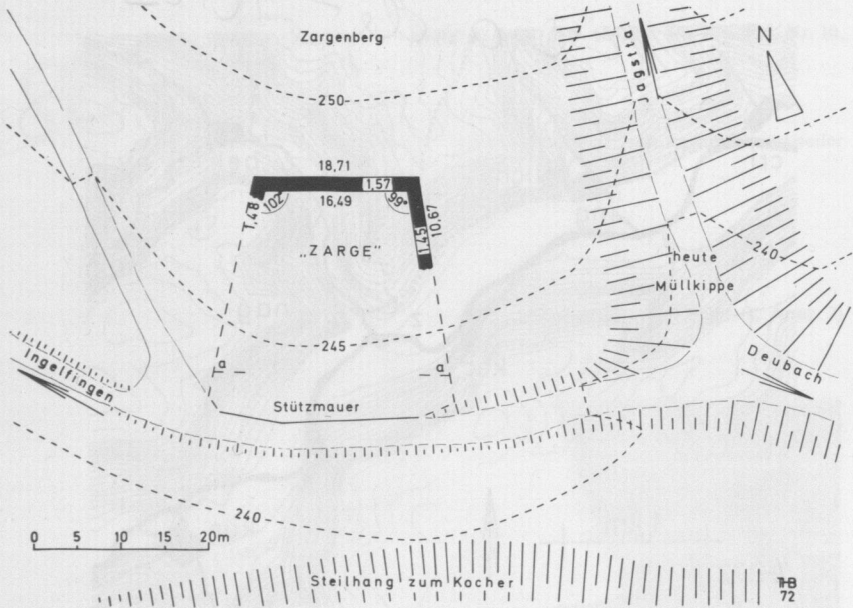
Abb. 2: Die „Zarge“, Grundriß.
