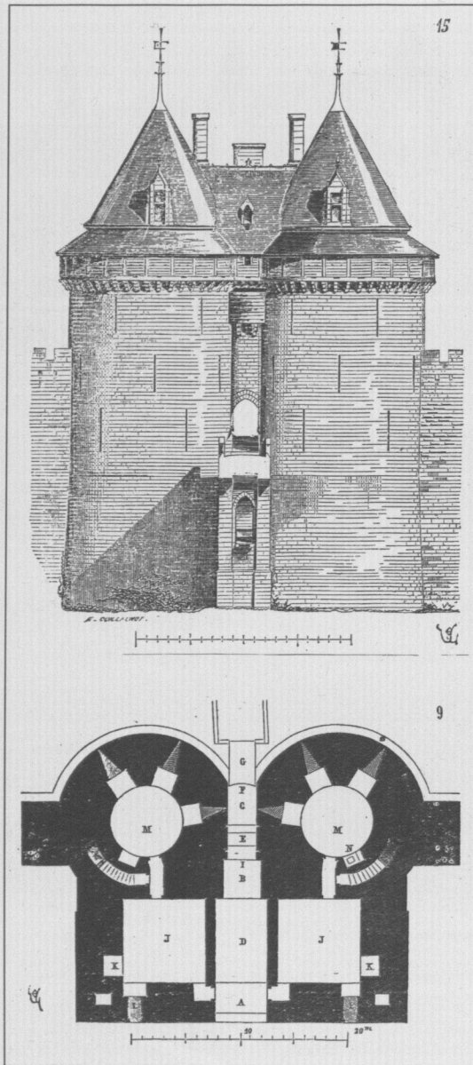
Abb. 3. Coucy (Dép. Aisne), "Porte de Laon", Rekonstruktionsversuch. Das im frühen 13. Jahrhundert entstandene Haupttor der Stadt war ein besonders monumentales Doppelturmtor aus der Epoche des Königs Philippe II. Auguste; solche Bauten hatten im 13. Jahrhundert begrenzte Wirkungen auch nach Deutschland.
