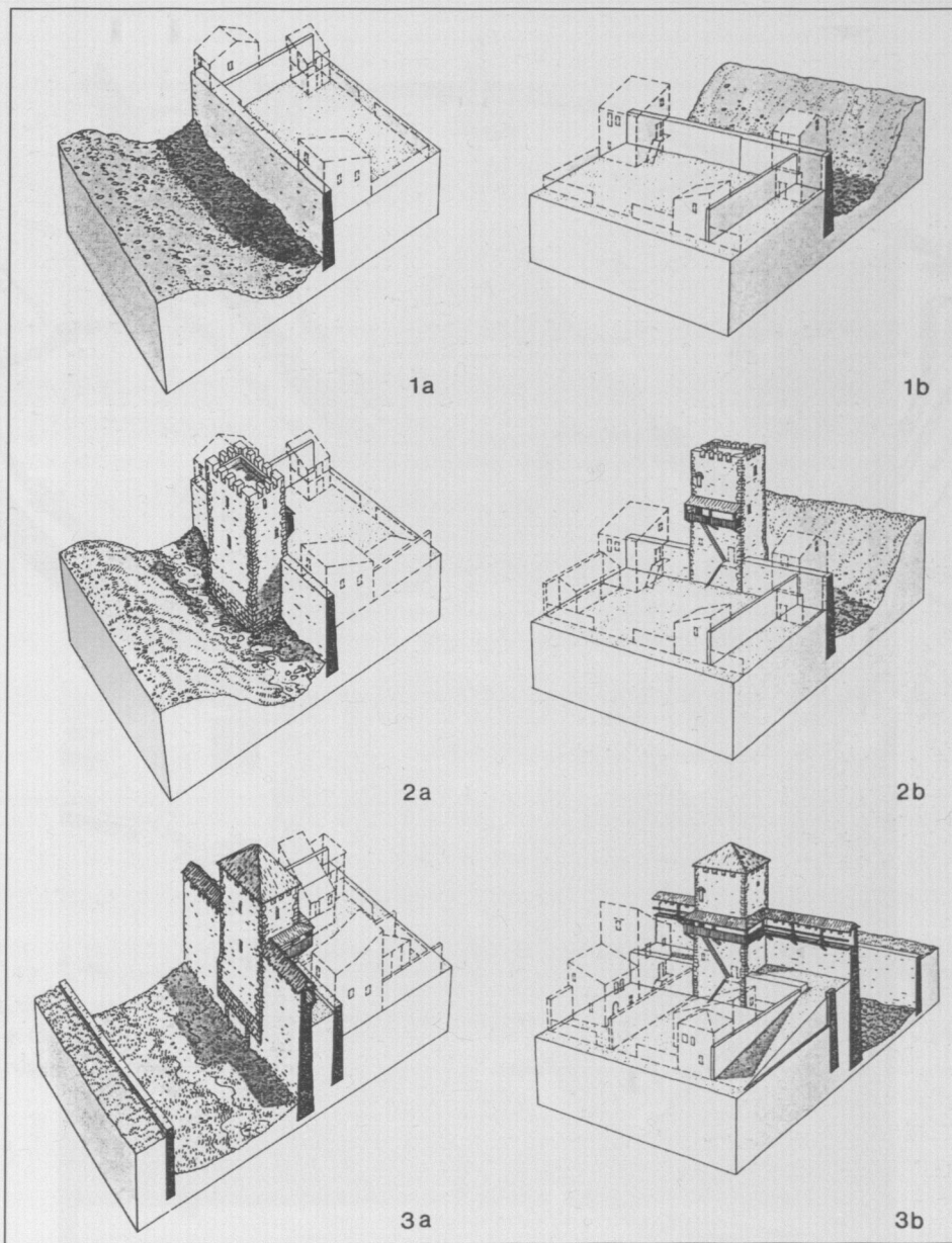
Abb. 10. Basel (Schweiz), Entwicklung der Stadtmauer am "Leonhardsgraben", nach den Ergebnissen von Archäologie und Bauforschung. Oben Zustand um 1100, in der Mitte gegen 1200, unten im 13. Jahrhundert; links jeweils von der Feldseite gesehen, rechts von der Stadt. (D'Aujourd'hui / Bing, Basler Zeitschrift ... , 1988; wie Anm. 1)
