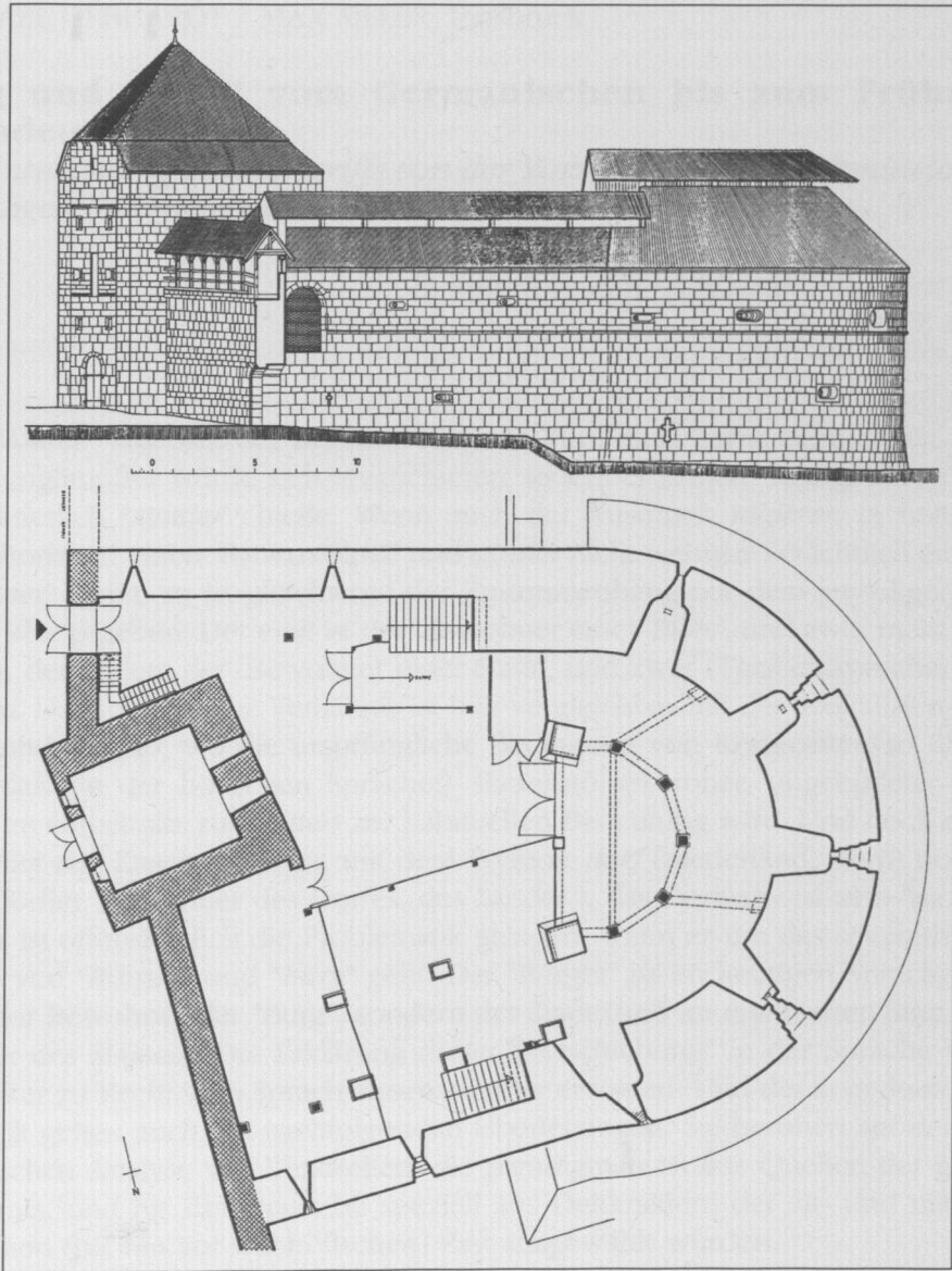
Abb. 20. Freiburg im Üechtland (Fribourg, Schweiz), "Großes Bollwerk". Das 1490-93 errichtete Werk ist das frühe Beispiel einer weitgehenden Anpassung an Artillerverwendung: flach und geräumig bot es dem Angreifer wenig Ziel, den Verteidigern Platz für viele Geschütze. Die in Italien entwickelten (Fünfeck-) Bastionen, die sich rund 50 Jahre später durchsetzten, verdrängten dieses Konzept durch sparsameren und effektiveren Einsatz der Geschütze. (Monuments d'Art et d'Histoire de la Suisse, Fribourg, I, 1964)
