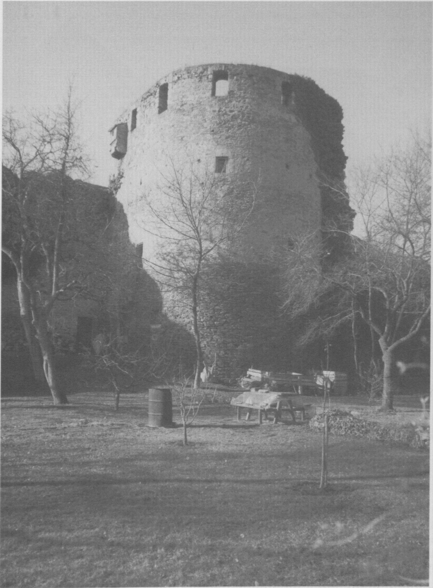
Abb. 18. Eggenburg (Niederösterreich), "Kanzlerturm". Um 1430 erbaut, ist der Turm ein Beispiel für den Beginn des Überganges zum Kanonenrondell: die Höhe ist reduziert, alle Scharfen sind Geschützscharten. Die Balkendecken waren jedoch noch ganz traditionsbezogen und wenig geschütztauglich.
