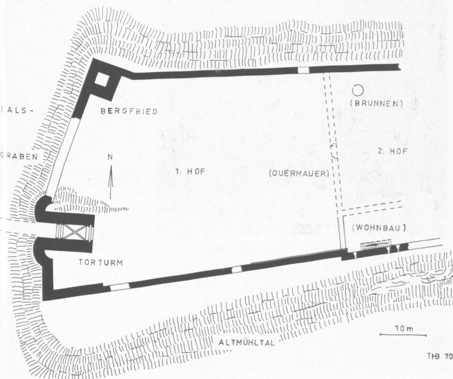
Abb. 2 Burg Hirschberg. Grundrißskizze des westl. Burgteiles: Türme und Schildmauer an der Angriffsfront, Wohnbau mit der vermuteten Quermauer. Rekonstruktion nach dem heutigen Bestand (unter Benutzung der Grundrisse im Inventar, Zeichnungen Abb. 2 u. 3 vom Verfasser)
