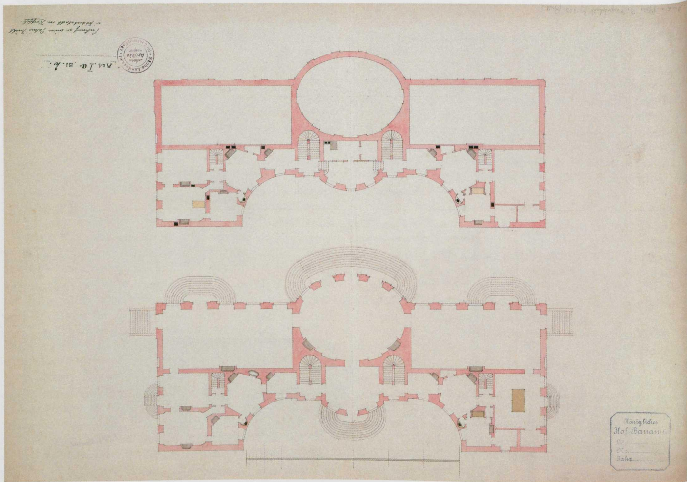
36. Friedrich August Krubsacius, Entwurf zum Grundriss des neuen Brühlschen Palais in Dresden-Friedrichstadt, um 1754 [Landesamt für Denkmalpflege Sachsen, Plansammlung M14 la Bl. 2]
