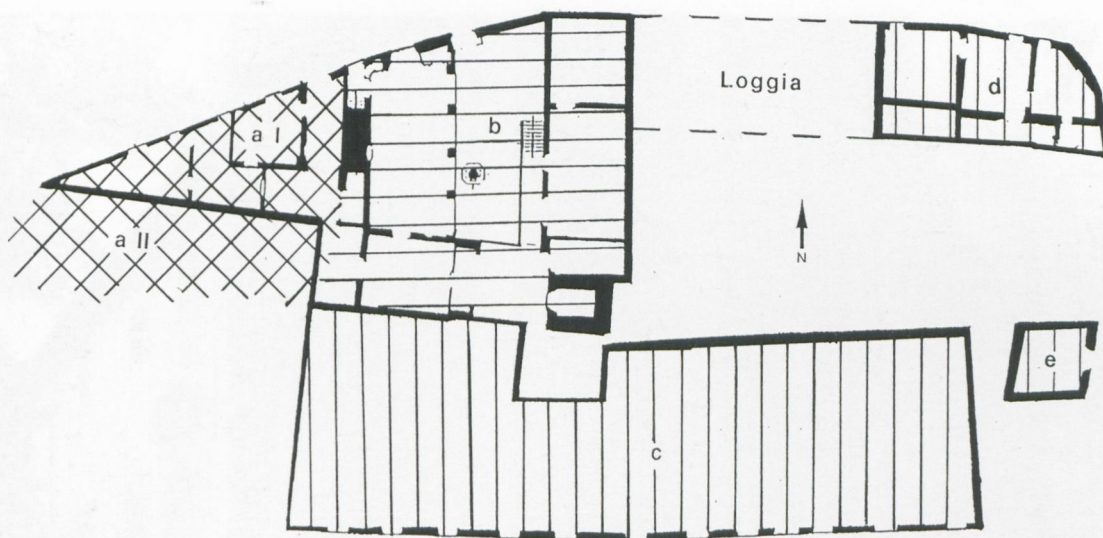
4 Montegufoni, Villa Acciaioli, Grundriß des Hauptgeschosses. Rekonstruktionsskizze der vorbarocken Bauzustände auf der Grundlage der Bauaufnahme von 1972; a I: 13./14. Jh. erhalten, a II: 13./14. Jh. überbaut?, b: um 1386, c, d, e: 15./16. Jh. (Wandöffnungen sind nur eingezeichnet, wenn sie erkennbar aus der betreffenden Zeit stammen).
