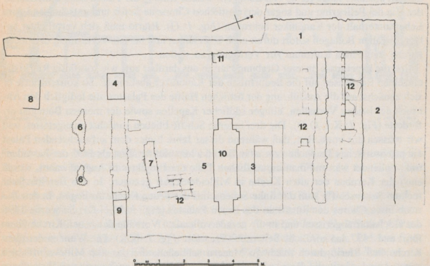
Fig. 2 Lageplan der Ausgrabung
