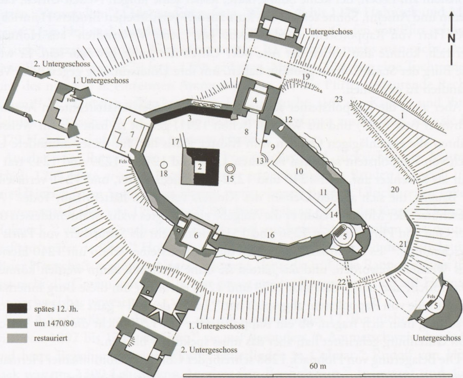
Abb. 2: Hohnack, Baualterplan auf der messtechnischen Grundlage der Senkrechtaufnahme bei Google Maps. Der „Kapellenturm“ (5) ist nicht so groß wie auf der Zeichnung von 1655 (Abb. 4), an der sich bisher fast alle neueren Grundrisszeichnungen orientierten.
