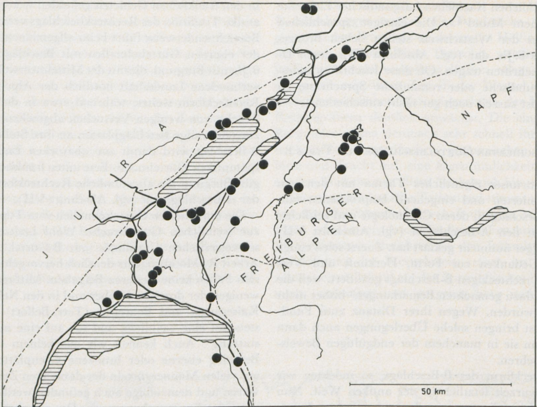
Abb. 4 Fundkarte mit der Verbreitung der tauschierten B-Beschläge in der Westschweiz (vgl. auch die Bem. auf S. 52)
