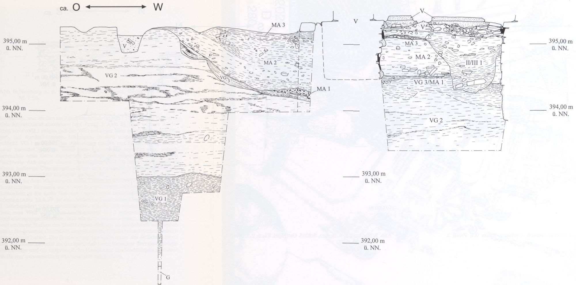
Abb. 3: Neuburg a. d. Donau, Schloß. Ostflügel, Räume 0.3/0.4, Profil 1. M. 1:50.
