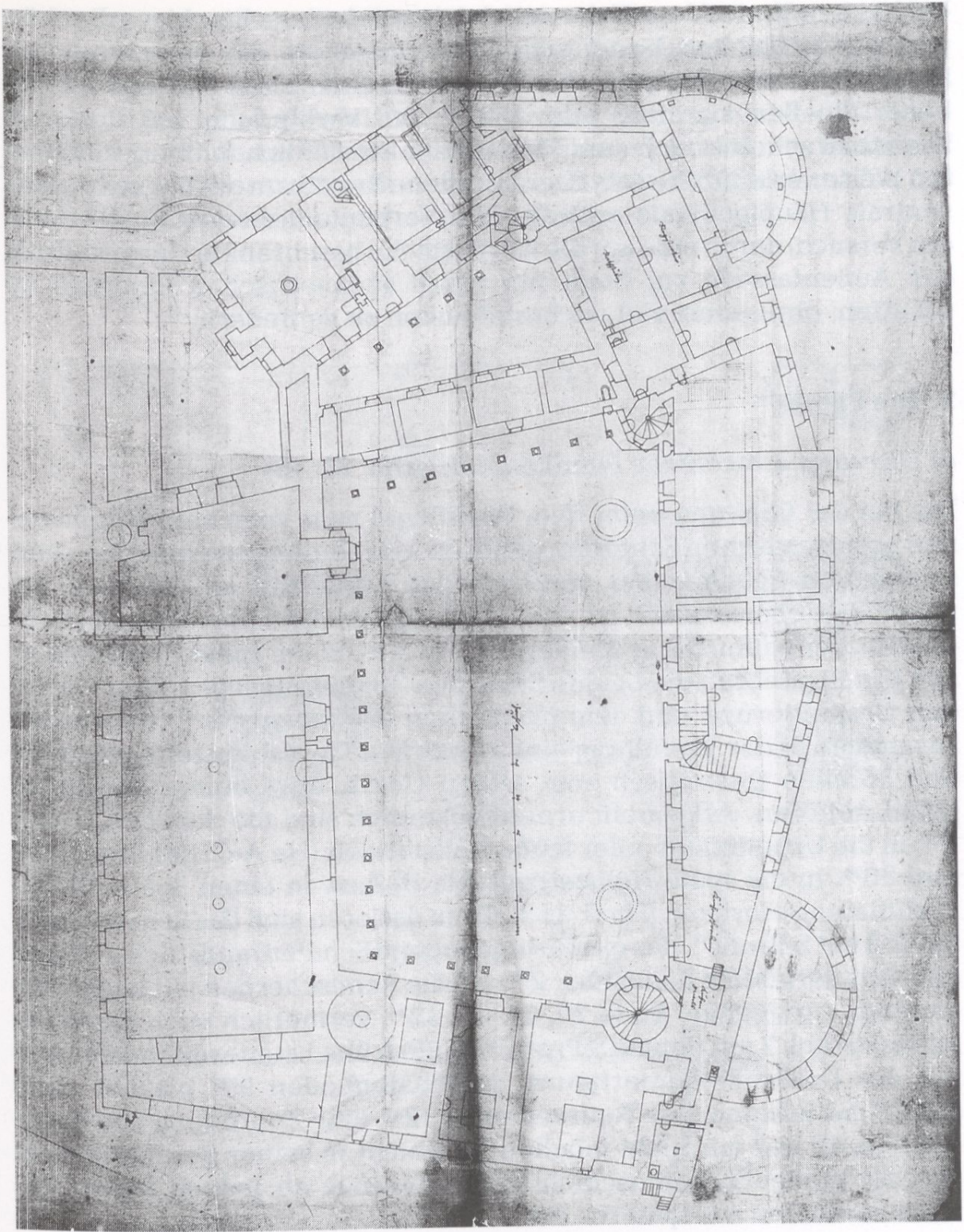
Abb. 14: Neuburg a. d. Donau, Schloß. Planzeichnung eines nicht ausgeführten Umbaus. Jeremias Doctor(?) um 1660 (HStA München, Plansammlung 3580).
