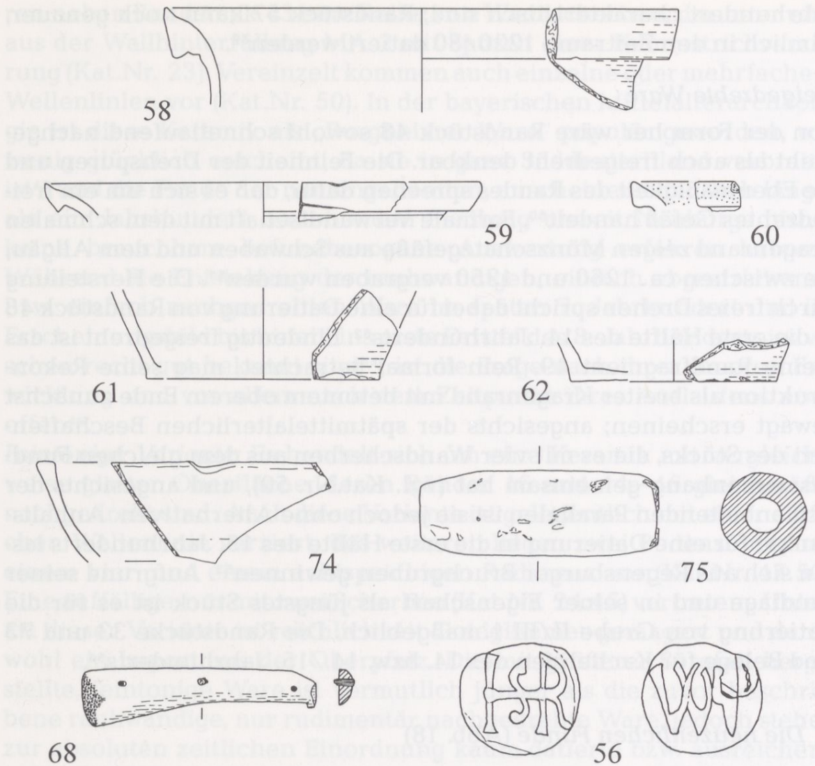
Abb. 18: Neuburg a.d. Donau, Schloß. Neuzeitliche Funde. 56 M. 1:1, sonst M. 1:3.
