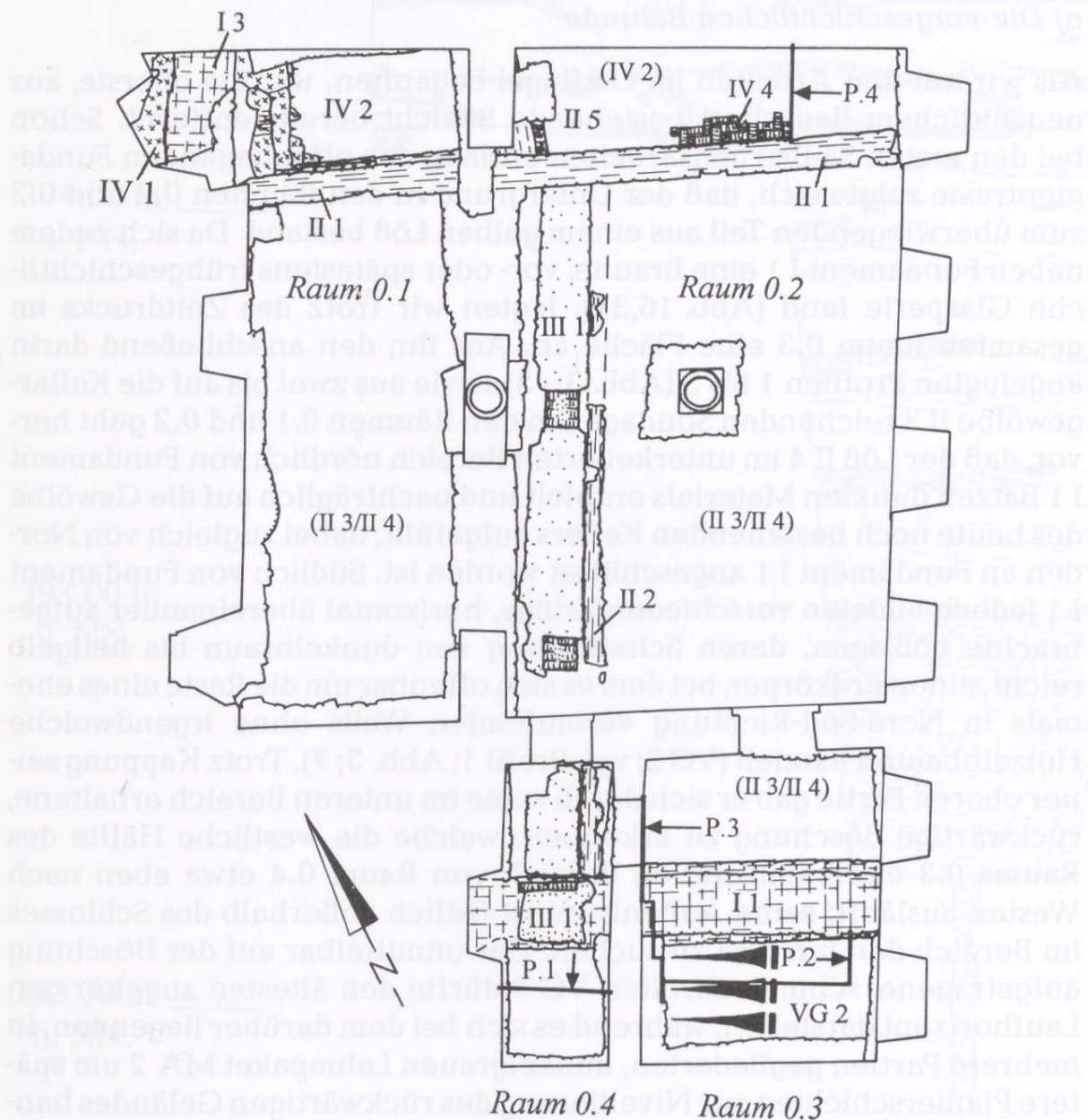
Abb. 2: Neuburg a.d. Donau, Schloß. Befundplan der Grabung 1994 im Ostflügel. — M. 1:200.
