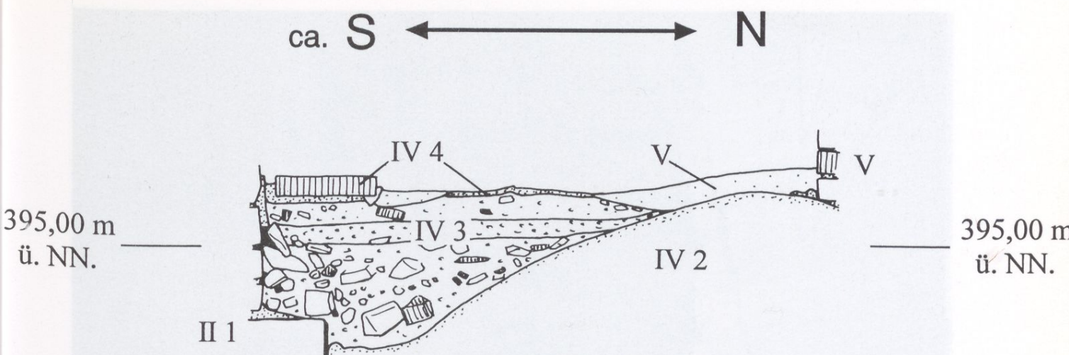
Abb. 6: Neuburg a. d. Donau, Schloß. Ostflügel, Raum 0.1, Profil 4. M. 1:50.
