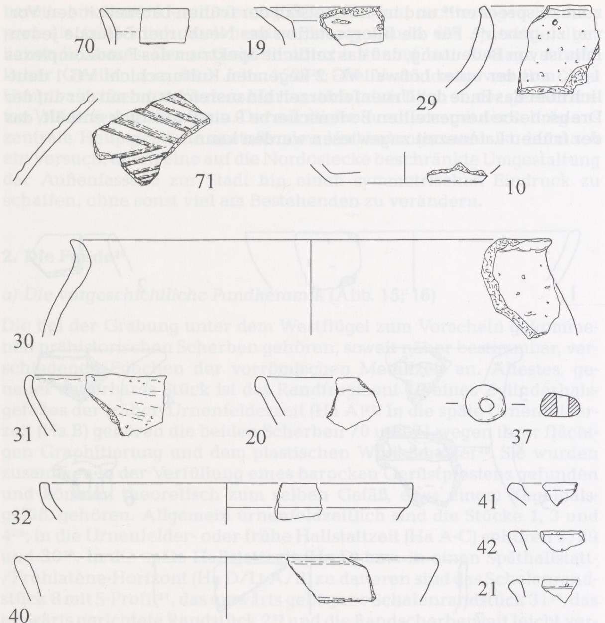
Abb. 16: Neuburg a.d. Donau, Schloß. Weitere vorgeschichtliche Funde. 37 M. 1:2, sonst M. 1:3.
