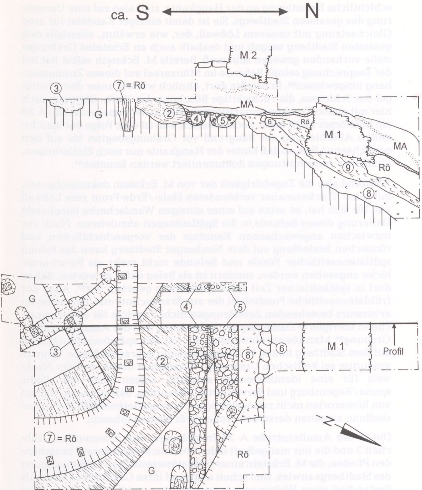
Abb. 20: Neuburg a. d. Donau. Profil und Planum der Ausgrabung in der Amalienstraße 26 A von 1963 (vereinfachte Umzeichnung nach Eckstein, Wehranlagen, Beilage I, A.C). Rö: römerzeitliche Befunde; MA: mittelalterliche Befunde. — M. 1:100.
