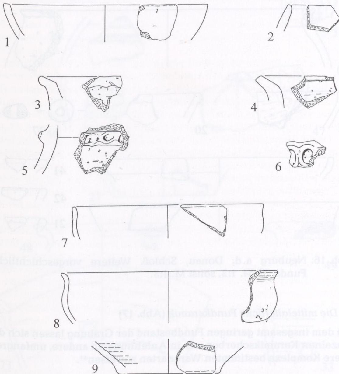
Abb. 15: Neuburg a.d. Donau, Schloß. Vorgeschichtliche Funde aus VG 1. M. 1:3.
