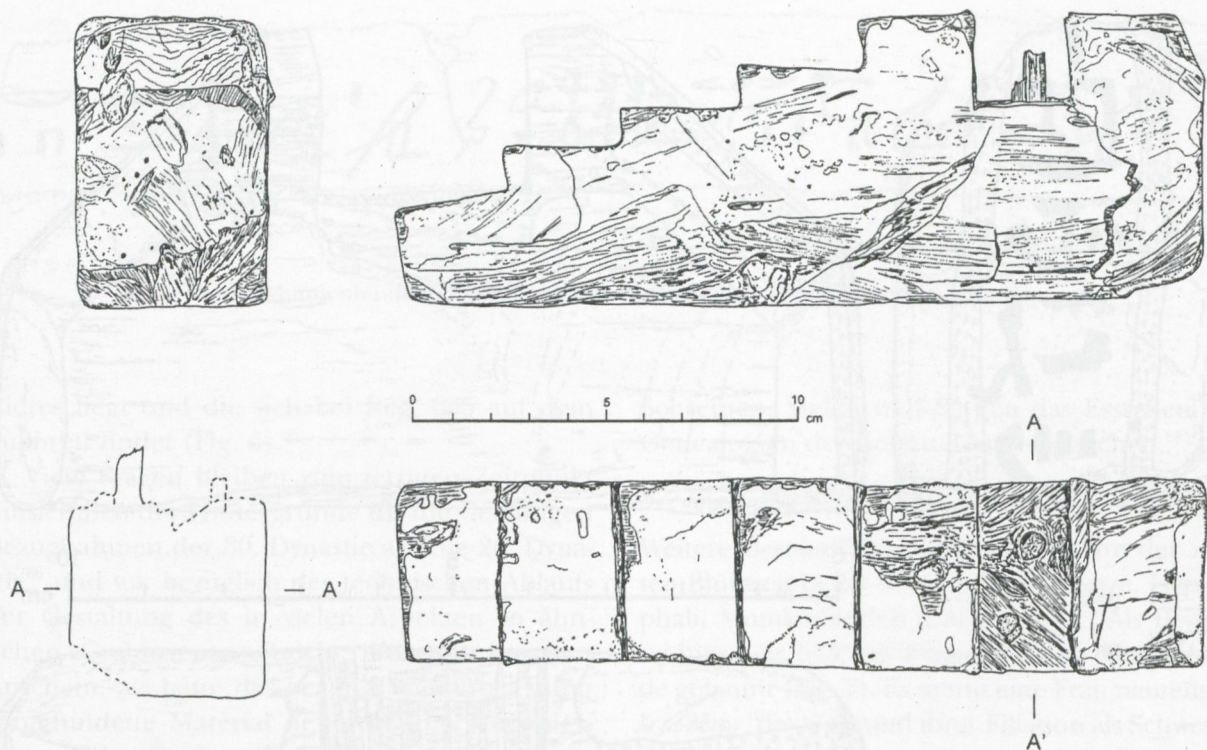
Fig. 9 Hölzerne Stelenhalterung K07/180.1 in Form einer Treppe (ptolemäisch) (Originalzeichnung: Zs. Thót, Umsetzung: J. Budka)
