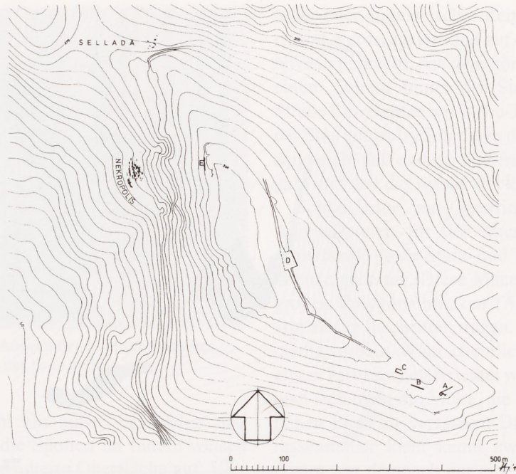
Abb. 4. Plan der noch erhaltenen und sichtbaren Bauten, Stützmauern und Straßen aus archaischer und klassischer Zeit
