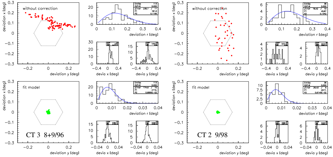
Abbildung 4.8: Die aus den Point Runs ermittelten Verschiebungsvektoren in der Kameraebene für die in Abb. 4.7 gezeigten Kalibrierungen. Jeder Punkt entspricht einem Point Run . In der oberen Hälfte der Abbildungen sind jeweils die Ergebnisse der Kalibrationsmessungen gezeigt; das Sechseck deutet die Abmessungen des zentralen Pixels an. Unten wurde in der Analyse der Point Runs bereits die Ausrichtungskalibration angewendet. Die verbleibenden Fehlansrichtungen (Residuen) sind ein Maß für die Genauigkeit der Kalibration; sie beträgt 0^{\circ}007 in radialer Richtung bzw. 0^{\circ}005 pro Achse.
