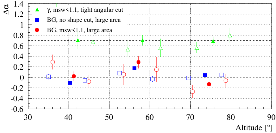
Abbildung 10.2: Ergebnisse der Vergleiche der Rohspektren von Mrk 501 und dem Krebsnebel als Funktion des untersuchten Zenitwinkelbereichs. Die gefüllten Symbole entsprechen den Ergebnissen der Zenitwinkelabschnitte 0^\circ - 25^\circ , 25^\circ - 40^\circ und 40^\circ - 60^\circ . Außerdem wurden diese Zenitwinkelabschnitte noch einmal halbiert, die Ergebnisse sind als offene Symbole dargestellt. Die \gamma -Erwartungswerte (Dreiecke) stimmen im Rahmen der statistischen Fehler mit dem erwarteten Wert von \Delta\alpha \approx 0.7 überein. Zu weiteren Details siehe Text.
