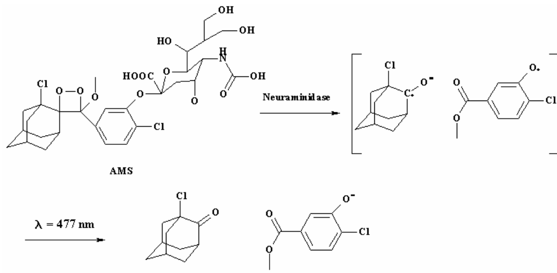
Abb. 2: Enzymatisch/chemisch induzierter Zerfall von AMS.
