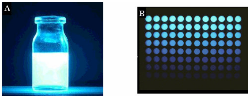
Abb 1.: Chemolumineszenz von AMS (A), Abhängigkeit der Lichtausbeute von AMS der Neuraminidasekonzentration in einem Mikrotiterplattenassay (B)
