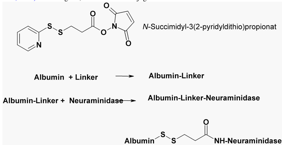
Abb. 11: Herstellung des Albumin-Neuraminidase-Konjugates
