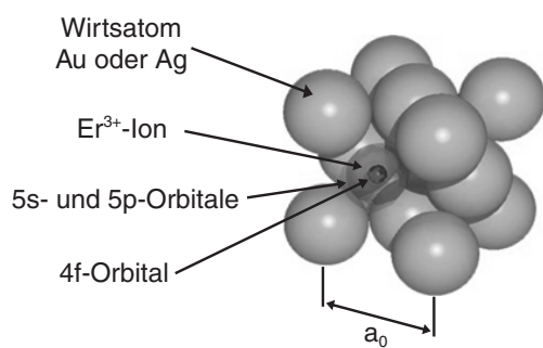
Abbildung 3.1: Ausschnitt aus der Gitterstruktur einer Au:Er - bzw. Ag:Er -Legierung in schematischer Darstellung. Die \text{Er}^{3+} -Ionen besetzen dabei reguläre Gitterplätze der fcc-Matrix des Wirtsmaterials. Die Gitterkonstante a_0 besitzt für beide Legierungen einen Wert von etwa 4,08 \text{ \AA}
