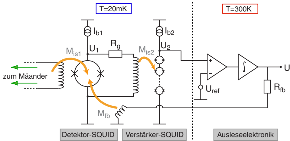
Abbildung 6.3: Schematische Darstellung der zweistufigen SQUID-Anordnung mit sich anschließender Rückkoppelschaltung. Als Verstärker-SQUID wird hier ein Serien-SQUID-Array verwendet.
