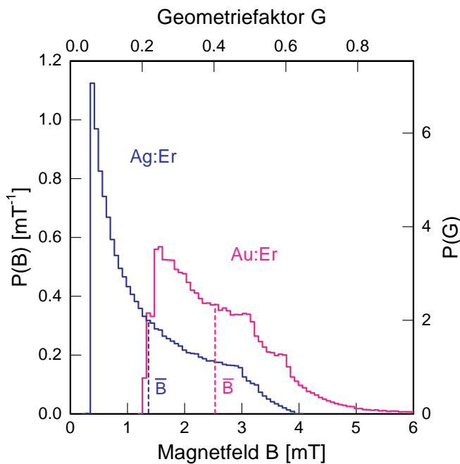
Abbildung 4.5: Häufigkeitsverteilungen der auftretenden Magnetfelder für die beiden im Rahmen dieser Arbeit untersuchten Aufbauten. Während die 3.5\ \mu\text{m} dicke Au:Er -Sensorschicht im Fall des Au:Er -Aufbau direkt auf dem Mäander aufgebracht war, wurde der 7,25\ \mu\text{m} dicke Ag:Er -Sensor aufgeklebt und ist folglich durch eine etwa 420\ \text{nm} dicke Klebeschicht vom Mäander getrennt. Es wurde hier von einem Dauerstrom von I_0 = 50\ \text{mA} ausgegangen.
