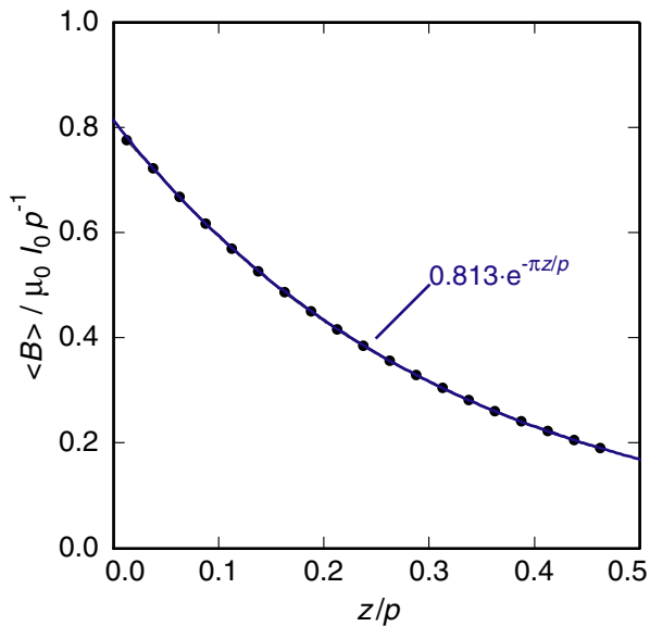
Abbildung 4.4: Betrag des mittleren Magnetfeldes einer sich im Abstand z über dem Mäander befindlichen dünnen Schicht als Funktion dieses Abstands. Der Nullpunkt des vertikalen Abstands wurde so gewählt, dass er mit der Oberfläche der isolierenden \text{SiO}_2 -Lage zusammenfällt, welche die mäanderförmige Detektionsspule bedeckt. Die Berechnung geht dabei von den gleichen Abmaßen für die Detektionsspule aus wie sie für die im Zusammenhang mit Abbildung 4.3 beschriebenen Anordnung angegeben wurden.
