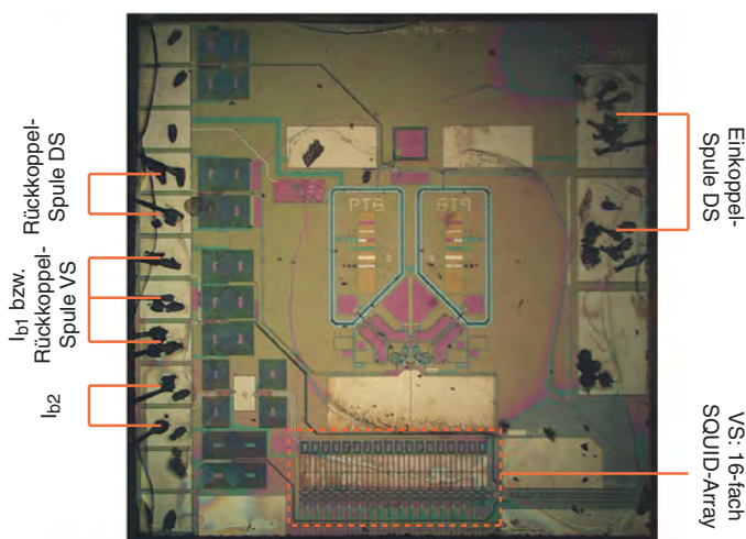
Abbildung 6.5: Genutzter SQUID-Chip im Fall des Ag:Er -Aufbaus. Auf dem Chip vom Typ C4XS116W sind sowohl das Detektor-SQUID (DS) als auch das Verstärker-SQUID (VS) integriert und bereits miteinander verschaltet. Als Verstärker-SQUID dient hier ein 16-fach SQUID-Array.
