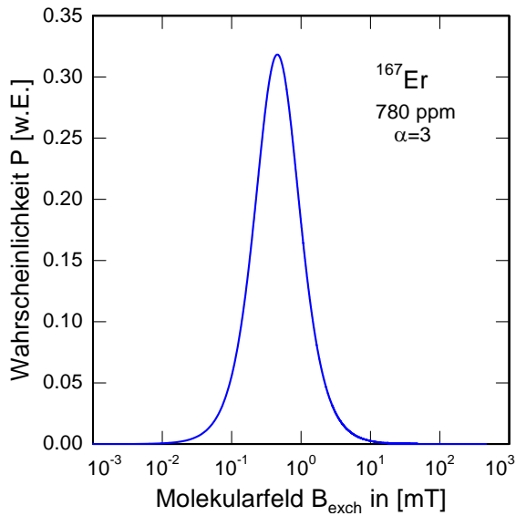
Abbildung 3.7: Verteilung der Molekularfelder für eine mit 780 ppm dotierte \text{Au:Er} -Probe. Für den Wechselwirkungsparameter der RKKY-Wechselwirkung wurde \alpha = 3 gewählt.
