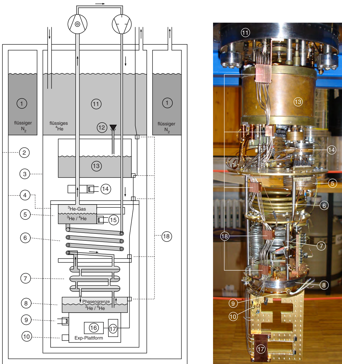
Abbildung 7.1: Aufbau des Mischkryostaten: (1) Stickstoff-Bad, (2) Äußerer Vakuumpotf, (3) Innere Vakuumpotf, (4) Strahlungsschilde, (5) Verdampfer/Still, (6) Kontinuierlicher Wärmetauscher, (7) Stufen-Wärmetauscher, (8) Mischkammer, (9) Mischkammer-Heizer, (10) Thermometer, (11) Helium-Bad, (12) Nadelventil, (13) 1K-Topf, (14) Film-Brenner, (15) Heizer für den Verdampfer, (16) Experiment, (17) Anschlussbox für die SQUIDS, (18) Thermische Ankoppungen für die in Cu/Ni-Kapillaren geführten SQUID-Zuleitungen
