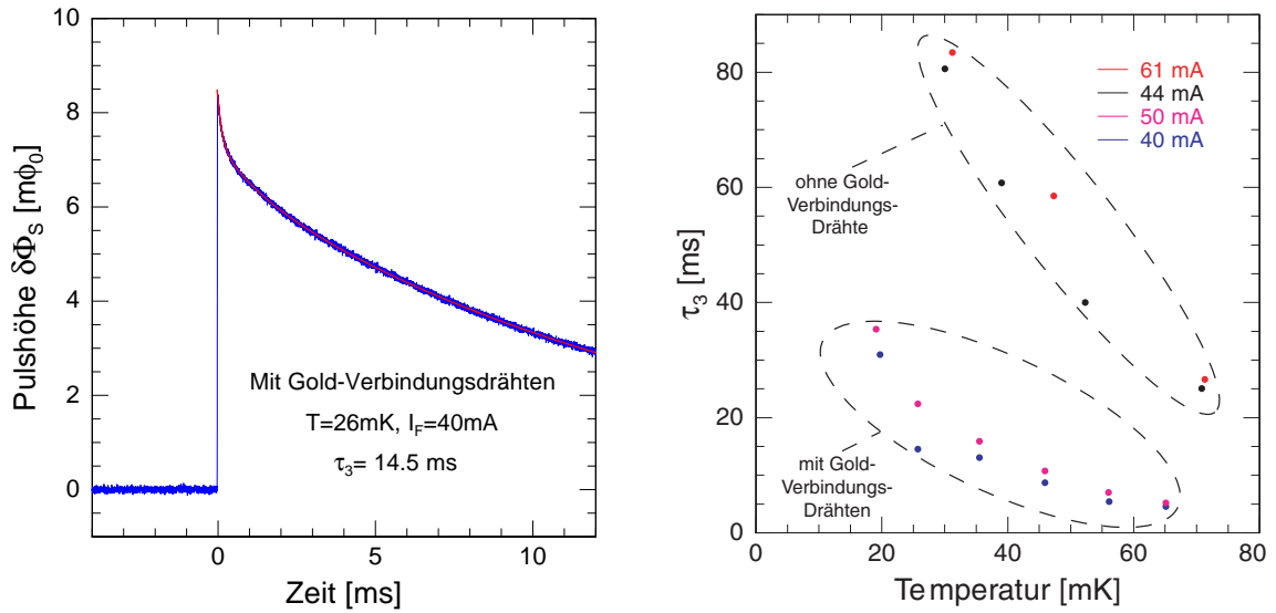
Abbildung 10.3: (links): Pulsantwort des über Gold-Drähte zusätzlich ans Wärmebad ange-koppelten Detektors bei der Absorption eines Röntgenquants mit einer Energie von 5,9 keV. Die Temperatur betrug 26 mK und der Feldstrom hatte einen Wert von 40 mA. (rechts): Tempe-raturabhängigkeit der Thermalisierungszeit \tau_3 für unterschiedliche Feldströme. Neben den Thermo-lisierungszeiten für den Detektor mit den Thermalisierungsverbindungen sind zum Vergleich auch die Thermalisierungszeiten für den Detektor ohne zusätzliche Thermalisierungsverbindungen gezeigt.
