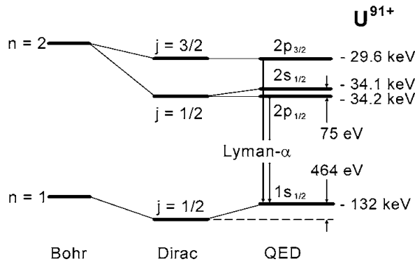
Abbildung 11.1: Energieschema für wasserstoffähnliches U^{91+} für die unterschiedlichen Atom-Modelle (aus [Ege05]). Die rechts daneben angegebenen Werte entsprechen den Bindungsenergien der Niveaus.
