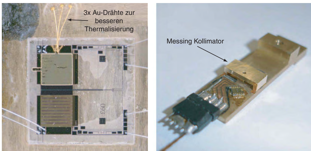
Abbildung 9.2: (links): Vergrößerung des Au :Er-Detektor-Chips. Neben den zur elektrischen Kontaktierung des Detektor-Chips verwendeten Aluminium-Drähten, ist der Sensor über 25 \mu\text{m} dicke und etwa 2 mm lange Gold-Drähte mit dem Messing-Halter verbunden. (rechts): Photographie des mit einem Messing-Kollimator versehenen Au :Er-Detektoraufbaus.
