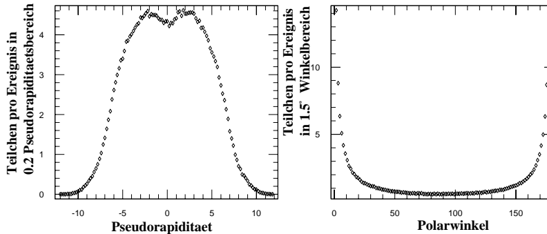
Abbildung 1.3: Die Teilchenanzahl pro Ereignis als Funktion der Pseudorapidität (links) und des Polarwinkels \theta (rechts). Die Kurven zeigen Ergebnisse einer Monte-Carlo Simulation.
