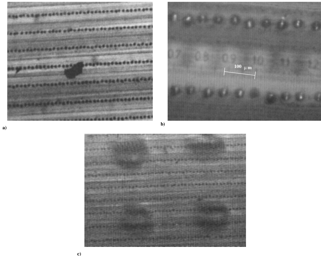
Abbildung 4.5: Mikroskopaufnahmen des Silikont Teppichs. Die dunklen Punkte stellen die Kanäle dar, die bei Druck einen leitenden Durchgang durch den Teppich ausbilden. In Aufnahme c) erkennt man die Fußabdrücke der PBGA-Kugeln.
