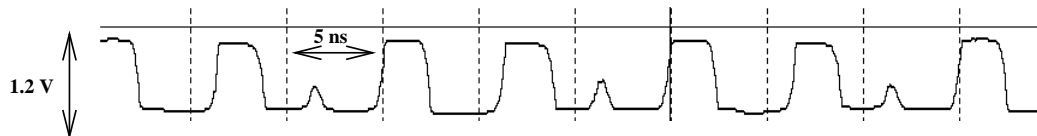
Abbildung B.4: Aufnahme eines 800 Mbit/s Signals mit dem Chip-Tester
