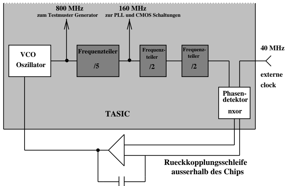
Abbildung 2.14: Blockschaltbild der PLL Implementation auf dem TASIC
