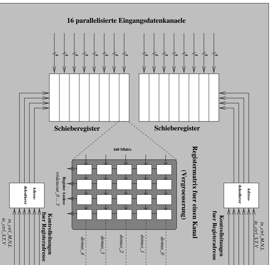
Abbildung 2.17: CMOS Schieberegister und Adreßdekodierer
