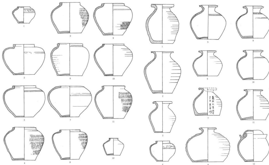
图四四〇 陶罐型式(1/5)
