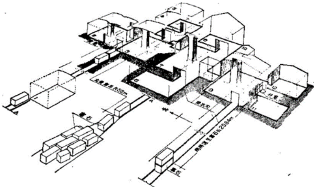
图二 龟山二号西汉崖洞墓透视图
