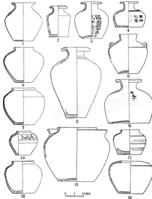
图一三 陶罐、瓶、罍
