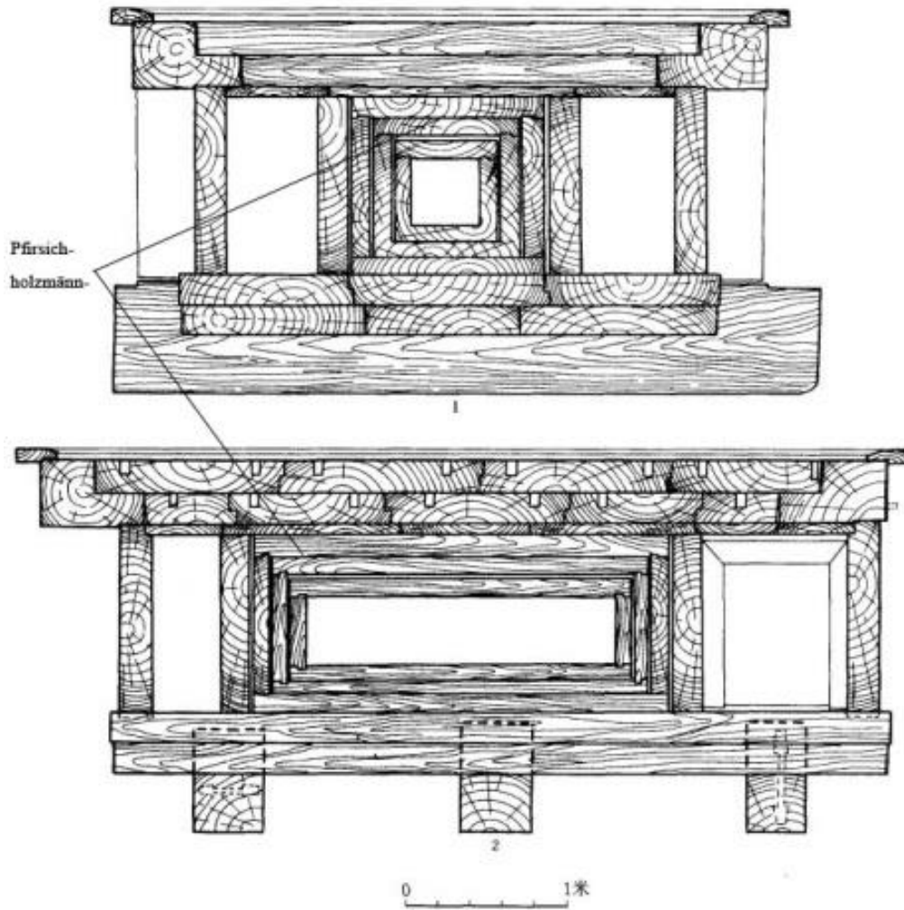
图一七 三号汉墓棺椁横、纵剖面图
