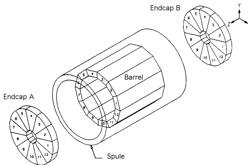
Abbildung 3.4: Aufbau des elektromagnetischen Kalorimeters.
