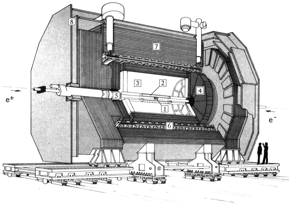
Abbildung 3.2: Der ALEPH-Detektor. 1 : Vertexdetektor, VDET. 2 : Innere Spurkammer, ITC. 3 : Zeitprojektionskammer, TPC. 4 : Elektromagnetisches Kalorimeter, ECAL. 5 : Luminositätskalorimeter, LCAL. 6 : Magnetspule. 7 : Hadronisches Kalorimeter, HCAL. 8 : Myonkammern.
