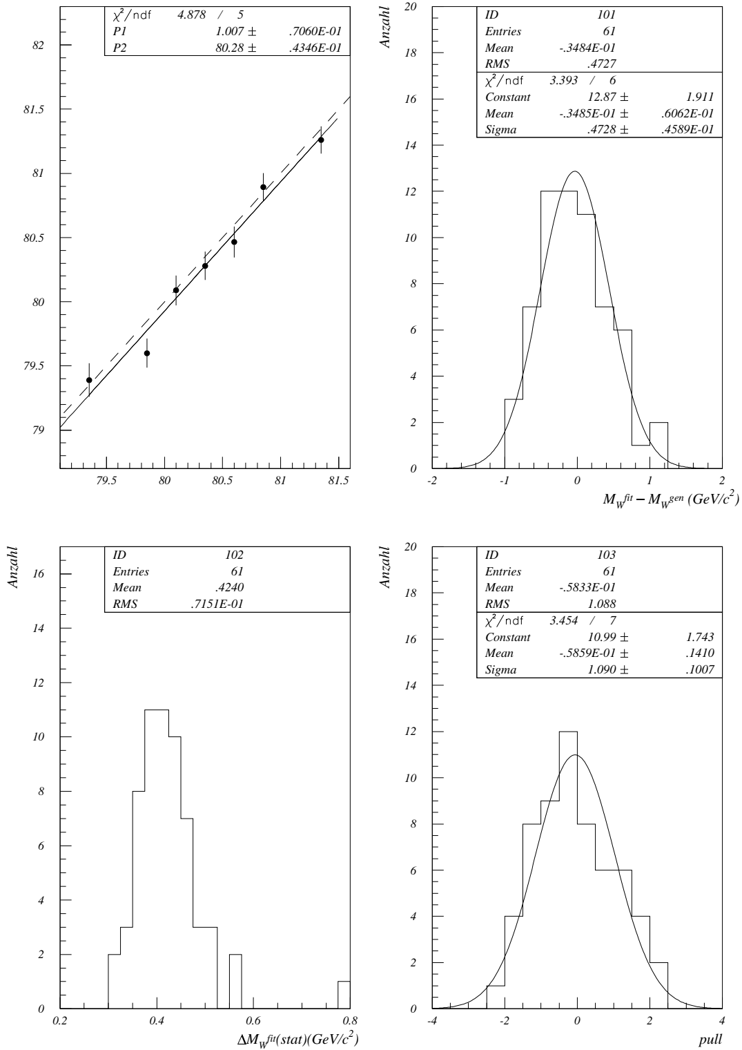
Abbildung 5.9: Kalibrationskurve (oben links), Massenauflösung (oben rechts), erwarteter Fehler (unten links) und Pullverteilung (unten rechts) bei einer Schwerpunktenenergie von 189 GeV.
