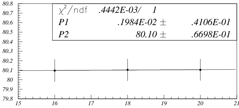
Abbildung 6.1: Abhängigkeit der gefitteten W -Masse vom Schnitt auf die Leptonenergie.
