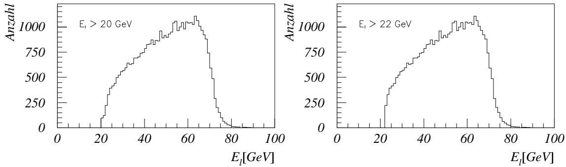
Abbildung 5.7: Vergleich der Leptonspektren bei verschiedenen Energieschnitten.
