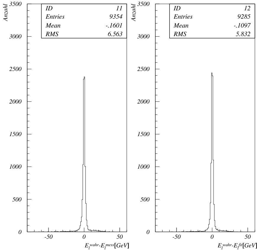
Abbildung 4.2: Leptonenergieauflösung vor (links) und nach (rechts) dem kinematischen Fit. Die Breite der Verteilung (RMS) ist durch den kinematischen Fit deutlich kleiner geworden.
