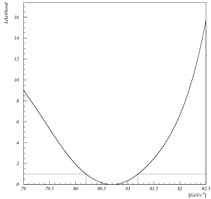
Abbildung 5.11: Likelihood in Abhängigkeit der W -Masse bei einer Schwerpunktenenergie von 189 GeV.
