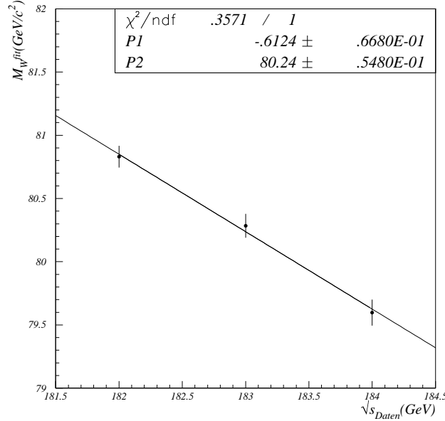
Abbildung 5.5: Abhängigkeit der gefitteten W -Masse von der in den Daten gewählten Schwerpunktenergie [9]. Es ist zu beachten, dass die hier benutzten Ereignisse keiner Detektorsimulation unterzogen wurden, da diese sehr lange Rechenzeiten in Anspruch nimmt. Dennoch erscheint es gerechtfertigt, die erhaltene Abhängigkeit M_W^{\text{fit}}(\sqrt{s}_{\text{Daten}}) auch auf den Fall von richtigen Daten zu übertragen.
