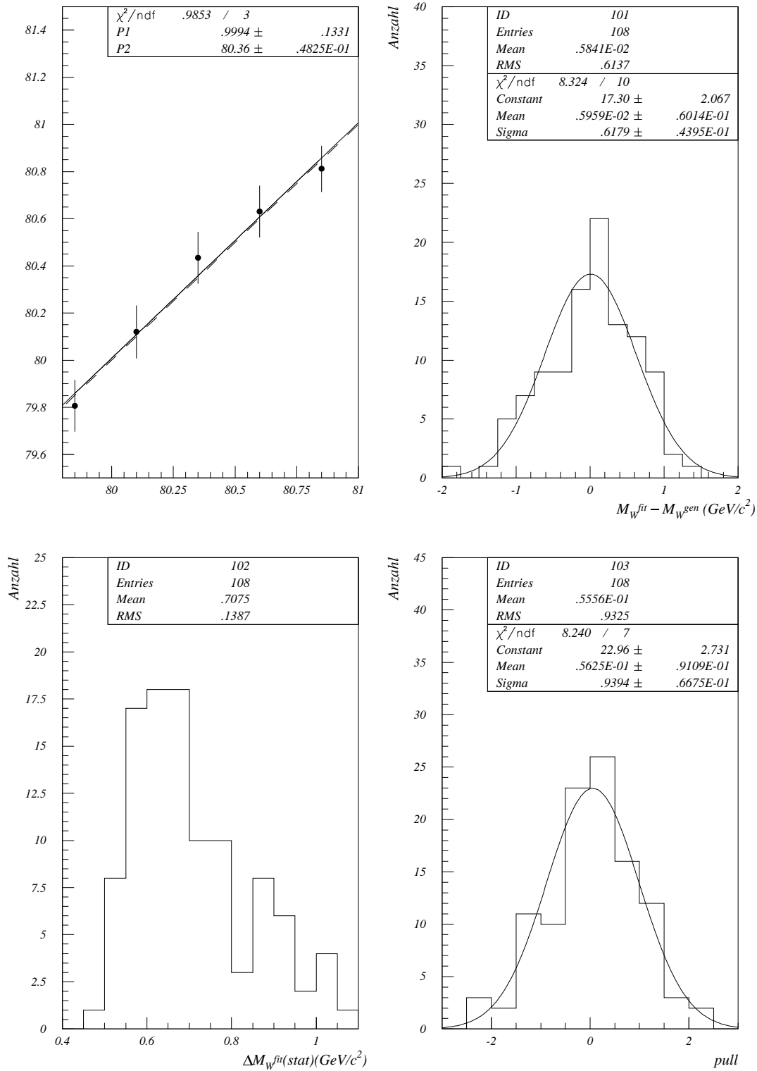
Abbildung 5.1: Kalibrationskurve (oben links), Massenauflösung (oben rechts), erwarteter Fehler (unten links) und Pullverteilung (unten rechts) bei einer Schwerpunktennergie von 183 GeV (semileptonischer Kanal). Alle benutzten Ereignisse durchliefen vor dem Massenfit einen 1C-Fit.
