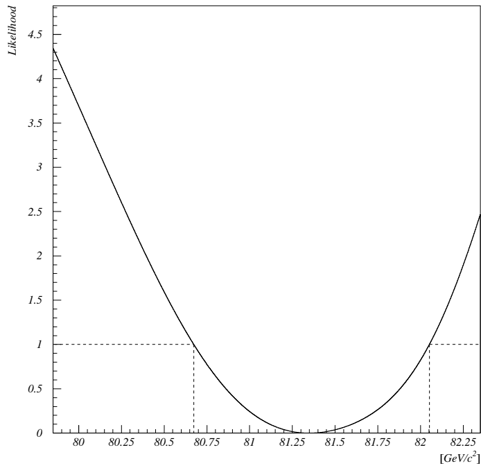
Abbildung 5.4: Likelihood in Abhängigkeit der W -Masse bei einer Schwerpunktenenergie von 183 \text{ GeV} .
