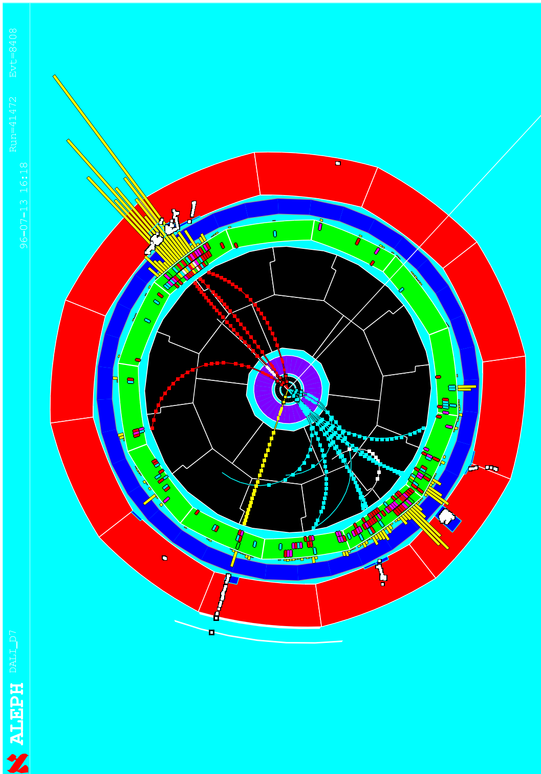
Abbildung 3.5: Beispiel eines semileptonischen WW -Ereignisses, das mit dem ALEPH-Detektor bei einer Schwerpunktennergie von 172 \text{ GeV} aufgenommen wurde. Zu sehen sind zwei Jets und ein Myon. Kennzeichnend wurde auch die Richtung des fehlenden Impulses, der einem Neutrino zugeschrieben wird.
