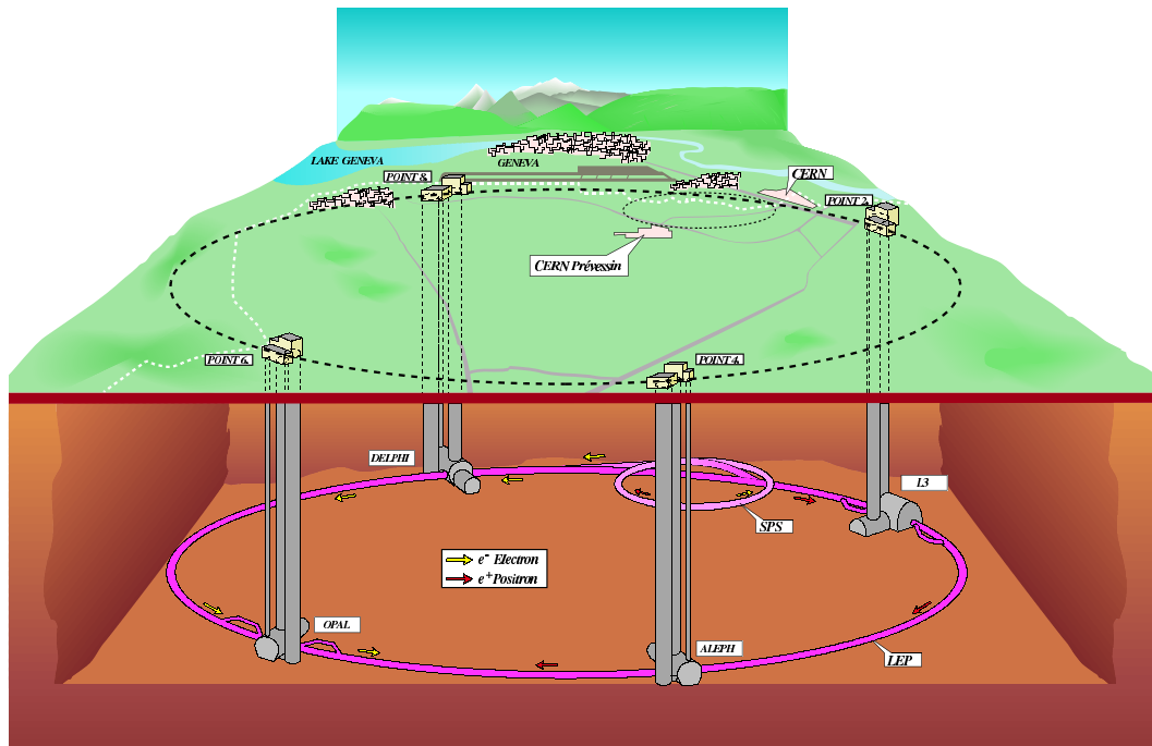
Abbildung 3.1: Der LEP-Ring.
