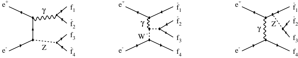
Abbildung 2.4: Beispiele für Nicht-CC03-Graphen, die zu 4 Fermionen im Endzustand führen.
