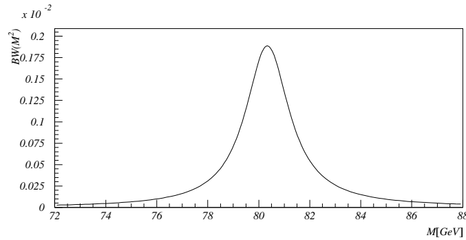
Abbildung 2.3: Das Massenspektrum des W -Bosons ist Breit-Wigner-verteilt. Die hier eingestellten Parameter sind M_W = 80.35 \text{ GeV}/c^2 und \Gamma_W = 2.1 \text{ GeV} .
