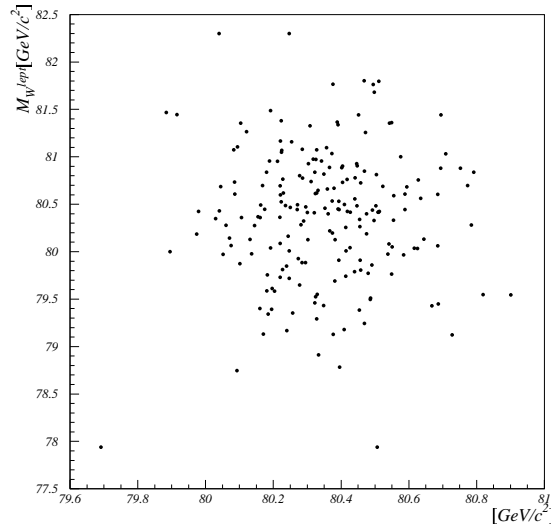
Abbildung 5.6: Für die Korrelation zwischen der offiziellen ALEPH-Analyse und der in dieser Arbeit benutzten Messmethode ergibt sich \rho = (2 \pm 5)\% .
