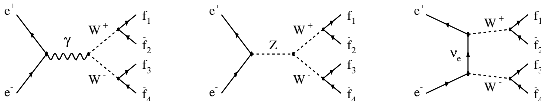
Abbildung 2.1: W -Paarproduktion durch CC03-Prozesse.
