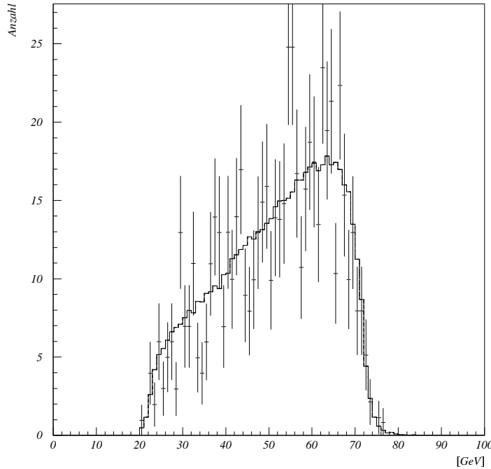
Abbildung 5.10: Leptonenenergiespektrum der Daten (nach Untergrundkorrektur) mit dem Referenzspektrum, das zur gefitteten W -Masse hin umgewichtet wurde, bei einer Schwerpunktsenergie von 189 \text{ GeV} .
