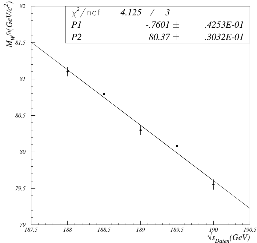
Abbildung 6.2: Abhängigkeit der gefitteten W -Masse von der in den Daten gewählten Schwerpunktenenergie bei \sqrt{s} \approx 189 GeV. Wie bei \sqrt{s} \approx 183 GeV (Abb. 5.5) wurden auch hier die Fermionimpulse auf Wahrheitsniveau benutzt, d. h. keine Detektorsimulation durchgeführt.
