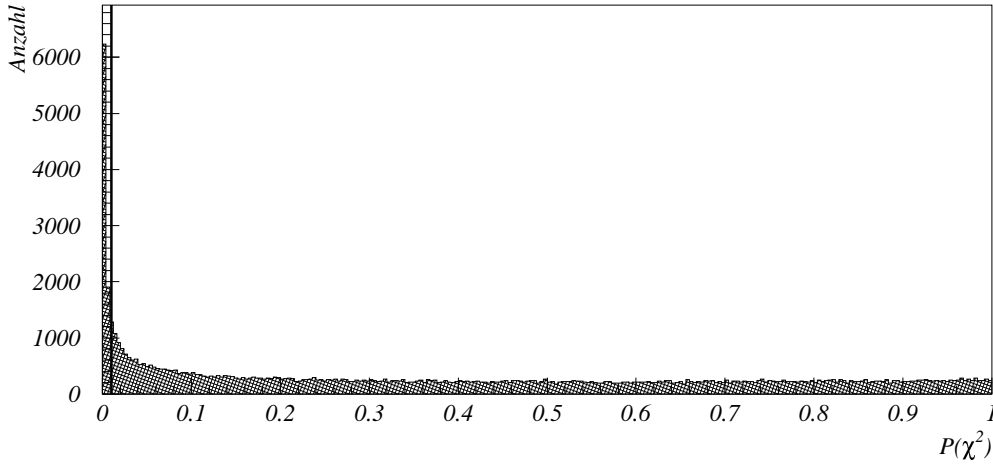
Abbildung 5.8: Die \chi^2 -Wahrscheinlichkeit ist im Idealfall flachverteilt. Um unerwünschte Ereignisse auszuklammern, wird auf die \chi^2 -Wahrscheinlichkeit bei 0.01 geschnitten.
