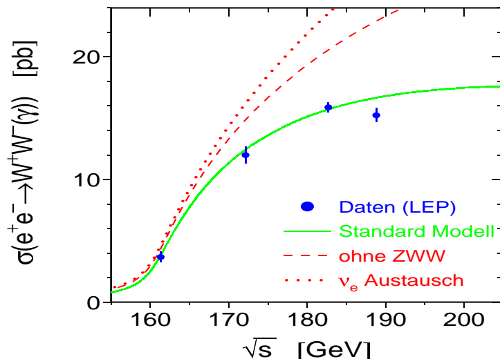
Abbildung 2.2: Anpassung des theoretischen totalen Wirkungsquerschnitts der W -Paarproduktion als Funktion der Schwerpunktsenergie im Rahmen des Standardmodells an die vorläufigen LEP-Daten ( W -Masse als freier Parameter) [7].
