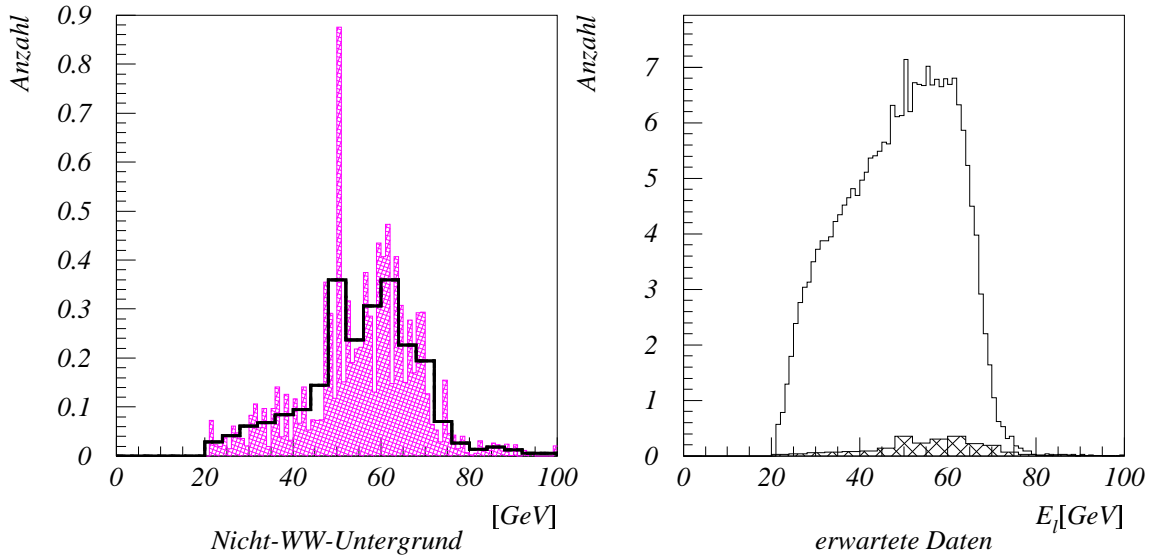
Abbildung 5.2: Energiespektrum des Nicht- WW -Untergrunds (links) und erwartetes Datenspektrum (rechts) nach Tab. 5.2. Der Anteil des Nicht- WW -Untergrunds aus dem linken Teilbild wurde im rechten Teilbild besonders gekennzeichnet.
