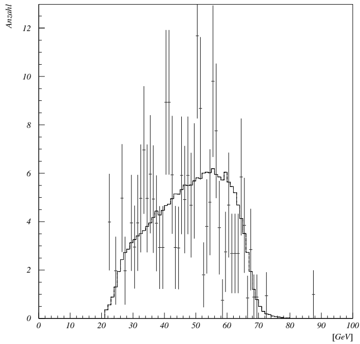
Abbildung 5.3: Leptonenergiespektrum der Daten mit umgewichtetem Referenzspektrum bei einer Schwerpunktenenergie von 183 \text{ GeV} .
