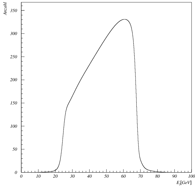
Abbildung 2.6: Energiespektrum des geladenen Leptons bei \sqrt{s} = 183 \text{ GeV} . Als Masse und Breite des W wurden hier 80.35 \text{ GeV}/c^2 bzw. 2.1 \text{ GeV} gewählt.
