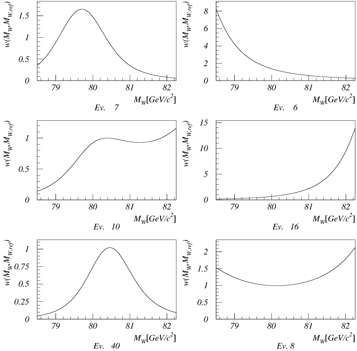
Abbildung 4.1: Gewicht w(M_W, M_{W,ref}) als Funktion von M_W für sechs ausgewählte Ereignisse. Die Masse, bei der diese generiert wurden, beträgt M_{W,ref} = 80.35 \text{ GeV}/c^2 .
